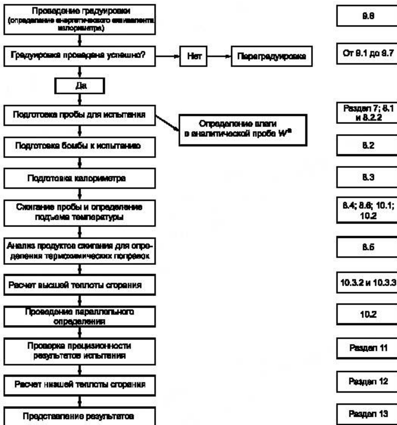
Рисунок G.1 — Схема рядового калориметрического испытания
