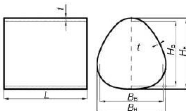
Рисунок А.2 – Вид трубы
