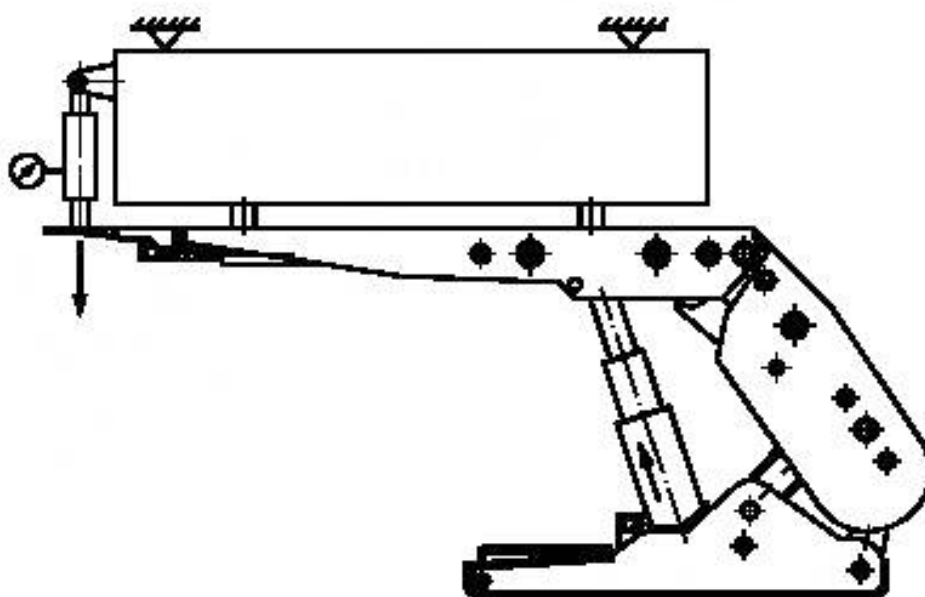
Рисунок В.4 — Схема нагружения для определения сопротивления на конце составной гидроподжимной консоли перекрытия
