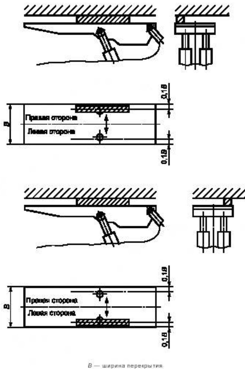
Рисунок Л.2 — Схемы испытаний на внецентренную нагрузку двухрядной секции крепи
