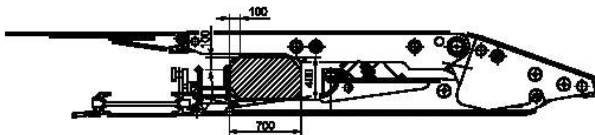
Рисунок 1 — Минимальные размеры прохода (размеры в мм)
