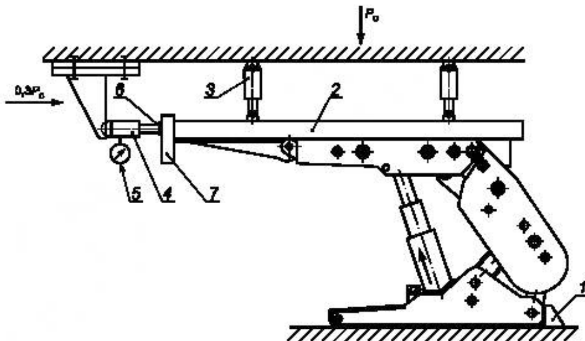
1 — упор; 2 — рама; 3, 4 — гидродомкраты; 5 — манометр; 6 — тензопора; 7 — упор
