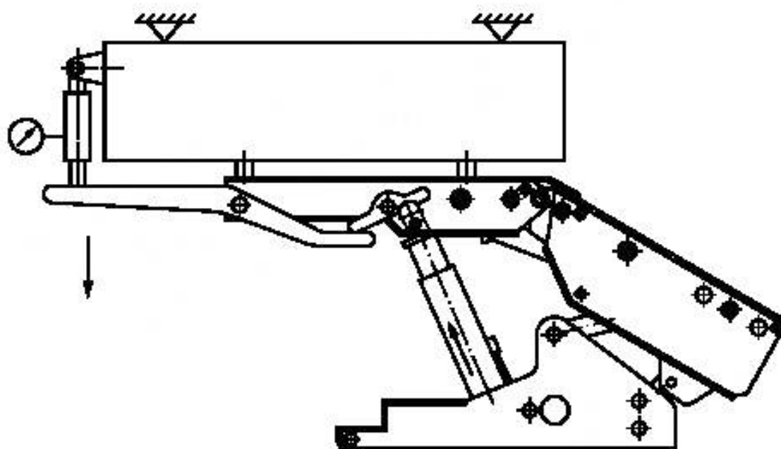
Рисунок В.6 — Схема нагружения для определения сопротивления на конце гидроподжимной консоли перекрытия рычажного типа
