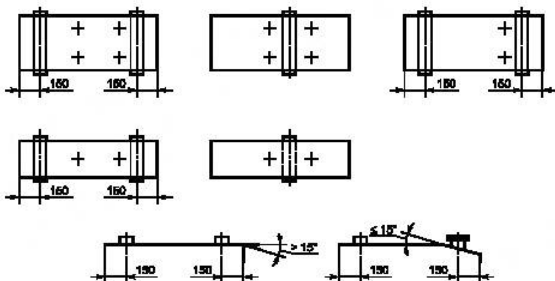
Рисунок Д.1 — Схемы нагружения перекрытий при испытании на изгиб
