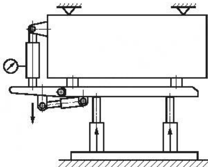
Рисунок В.3 — Схема нагружения для определения сопротивления на конце гидроподжимной консоли (козырька) перекрытия
