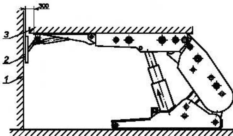
Рисунок И.1 — Схема нагружения механизма удержания забоя
