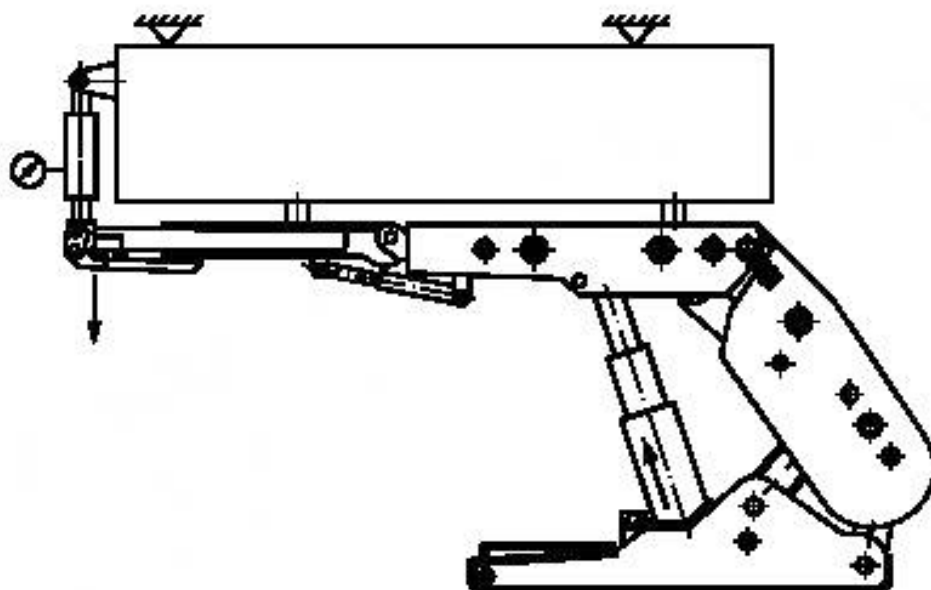
Рисунок В.5 — Схема нагружения для определения сопротивления на конце гидроподжимной консоли перекрытия пенального типа
