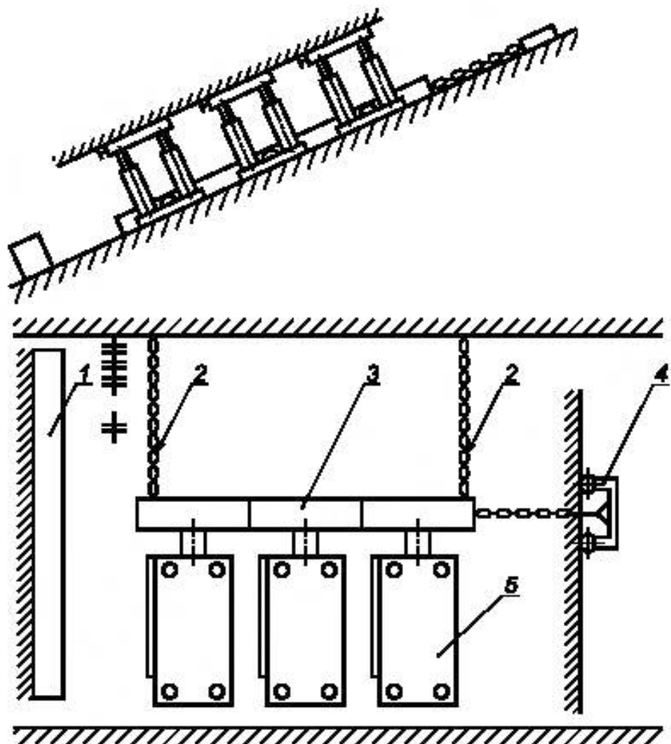
1 — страховочная балка; 2 — якорное устройство; 3 — став конвейера; 4 — тележка подвески; 5 — секция крепи
