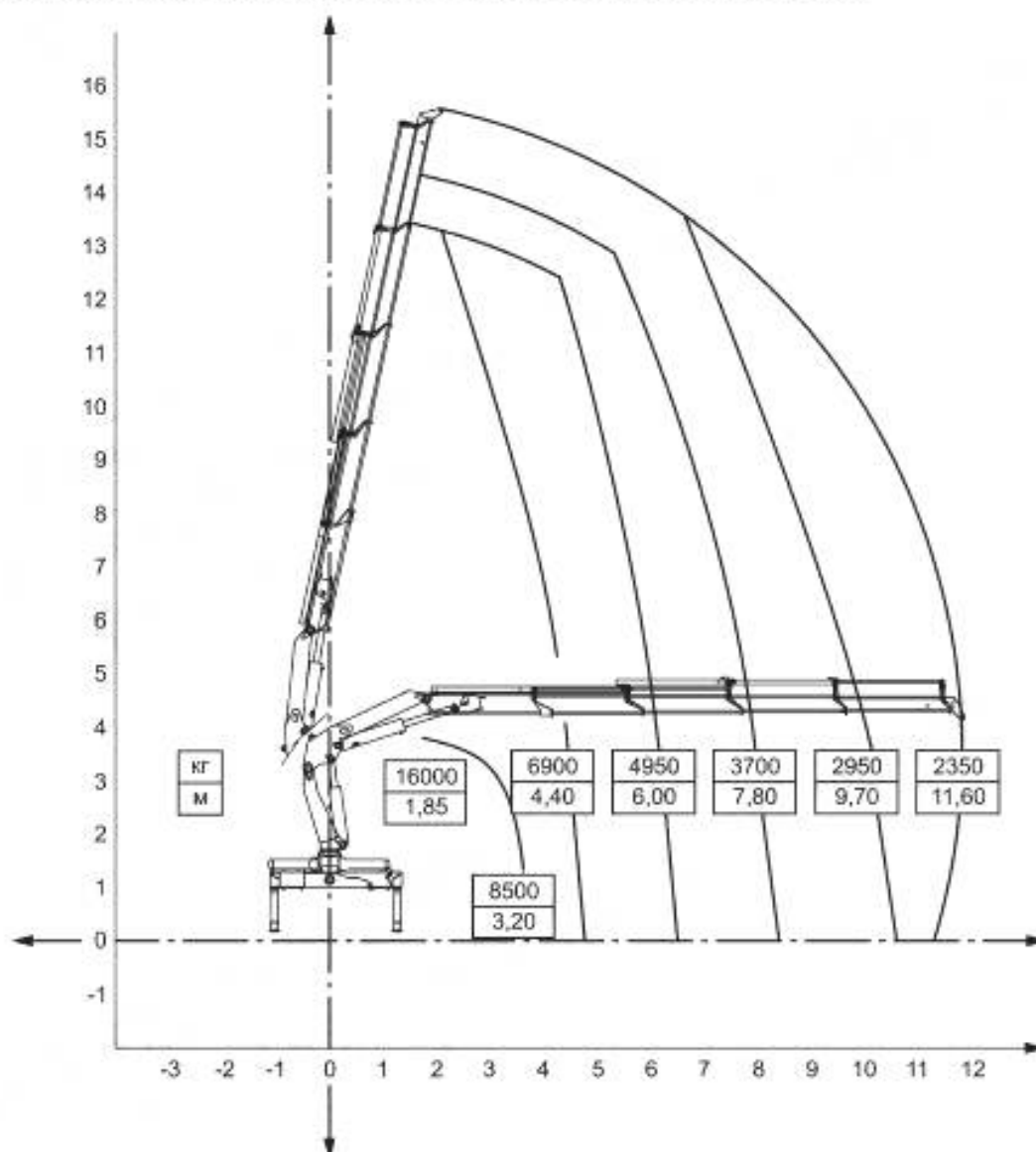
Рисунок 3 — Пример грузовой характеристики
