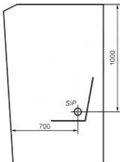
Рисунок В.1 — Минимальные внутренние размеры кабины
