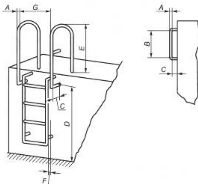
Рисунок А.1 — Перила и поручни
