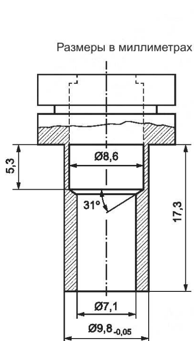
Рисунок А.4 — Рекомендуемые размеры втулки для устройства измерения температуры
