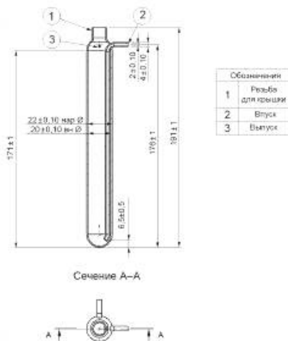
Рисунок А.3 — Испытательный сосуд
