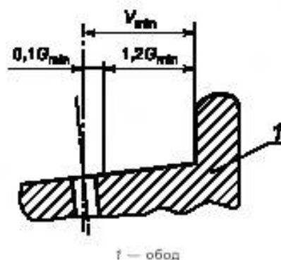
Рисунок 9 — Расположение отверстия для вентиля камерной шины
