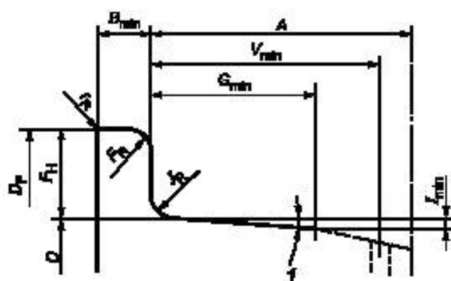
Рисунок 5 — Сечение посадочной полки
