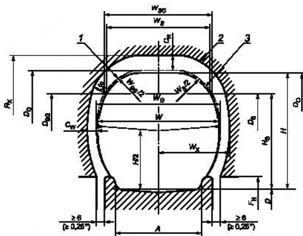
Рисунок 2 — Допуски на увеличение и на зазоры
