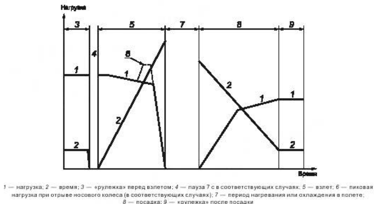
Рисунок 6 — Последовательность испытательного цикла — полный цикл испытания
