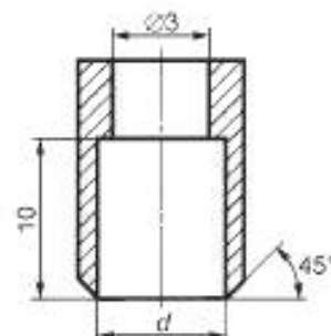
Исполнение II, применяемое для внутренних диаметров насадки более 3 мм
