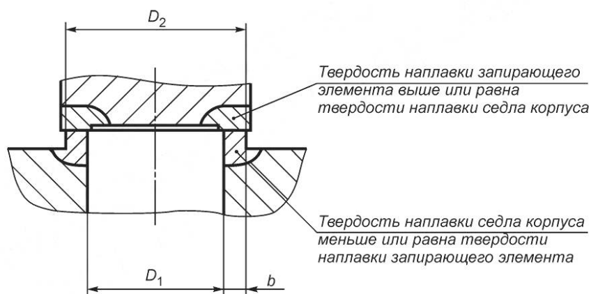
Рисунок Е.1 — Плоское уплотнение в затворе
