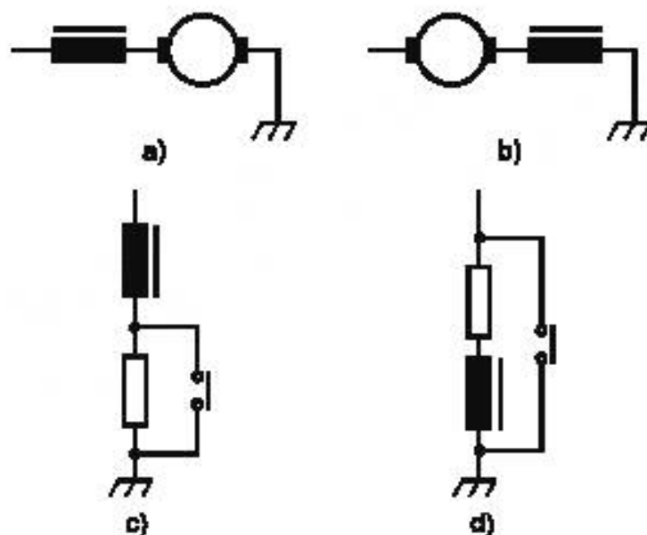
а) и б) — соединение обмотки возбуждения/якоря электродвигателя с последовательным возбуждением в) и г) — соединение при коротком замыкании имитируемой нагрузки
