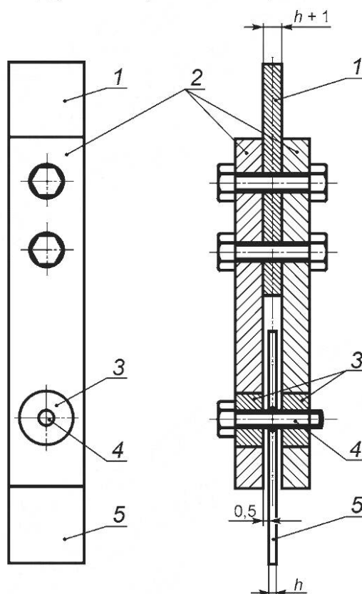
Рисунок Д.1 — Нагрузочные плиты и испытательная установка
