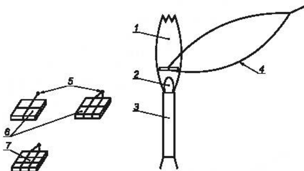
1 — факел пламени; 2 — восстановительная зона пламени; 3 — горелка Бунзена; 4 — пинцет; 5 — нихромовая проволока; 6 — образец, армированный однонаправленными углеродными волокнами; 7 — образец, армированный плетеной тканью из углеродного волокна
