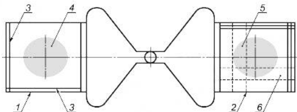
1 — полость 1; 2 — полость 2; 3 — линии разметки; 4 — зона испытания (диаметр 50 мм); 5 — п-образец; 6 — р-образец
