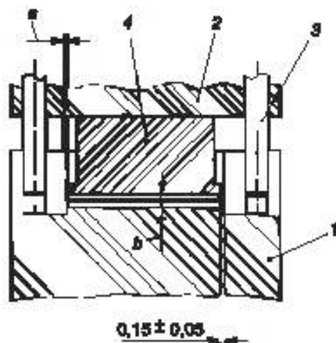
Рисунок 1 – Пресс для формования
