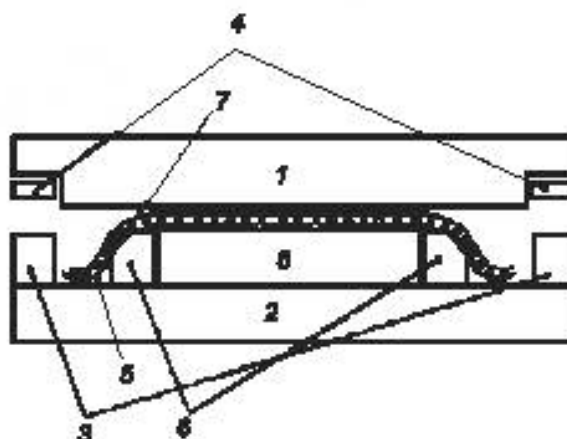
Рисунок 6 – Схема формирования пластин в мембранном прессе (вакуумный метод)
