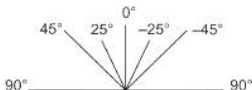
Рисунок А.1 – Углы, используемые для описания ориентации слоя в ламинате
