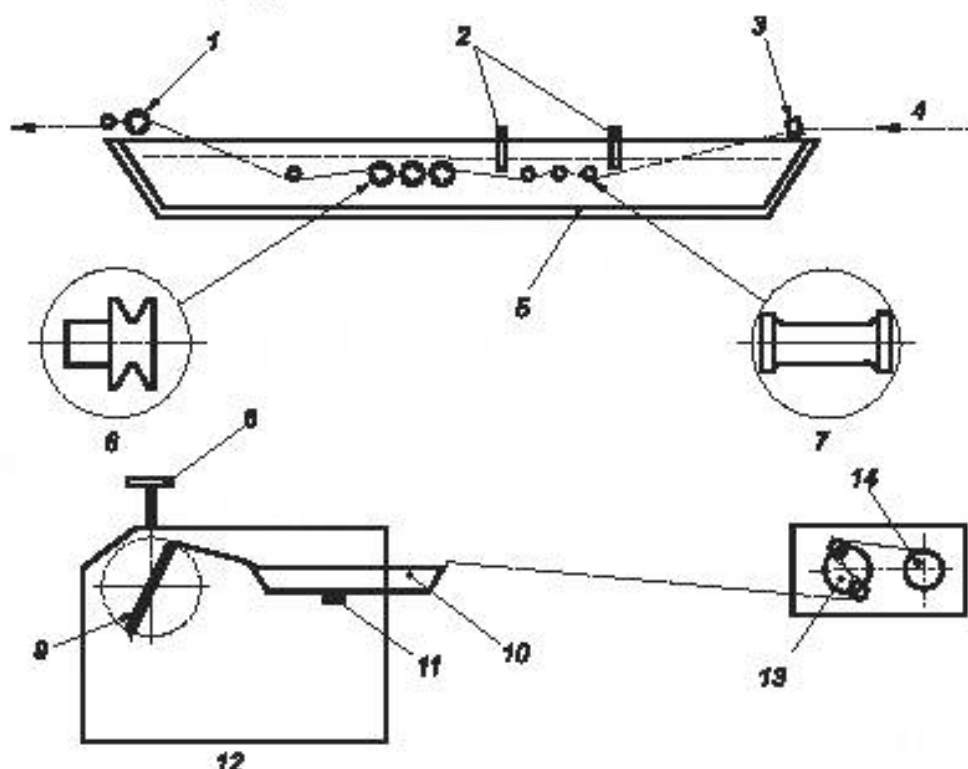
1 – приемный направляющий ролик; 2 – устройства для задержания пены; 3 – подающий направляющий ролик; 4 – ровинг; 5 – ванна для пропитки с двойными стенками; 6 – штанга нитеводителя с желобком; 7 – плоская штанга нитеводителя; 8 – теплоизлучающая панель; 9 – формообразующее устройство; 10 – ванна для пропитки; 11 – шарнирная рука; 12 – намоточная машина; 13 – система регулирования натяжения; 14 – бобина ровинга или упаковка
