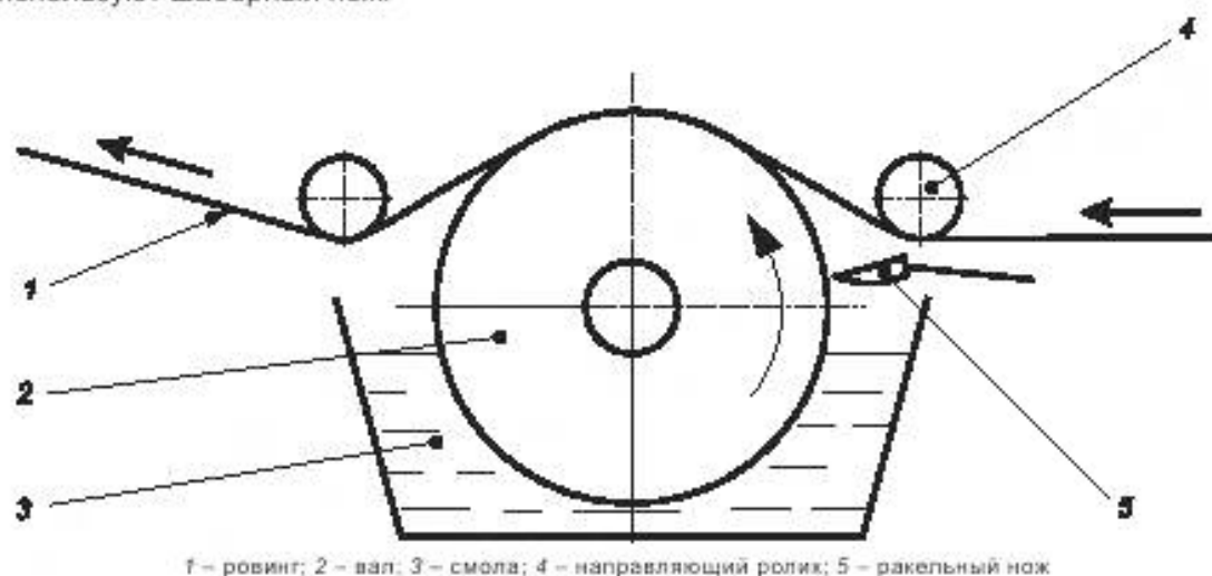
Рисунок 2 – Вал для пропитки
