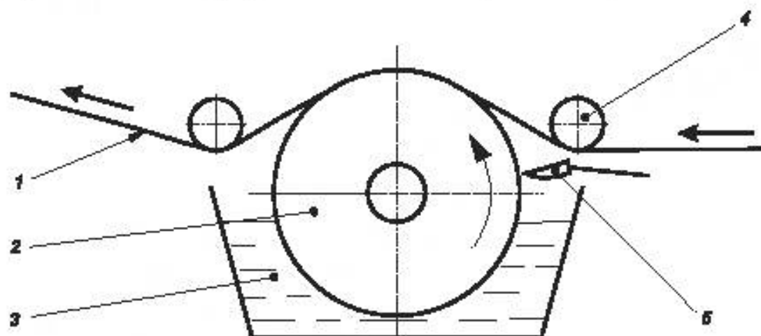
1 – ровинг; 2 – вал; 3 – смола; 4 – направляющий ролик; 5 – ракельный нож
