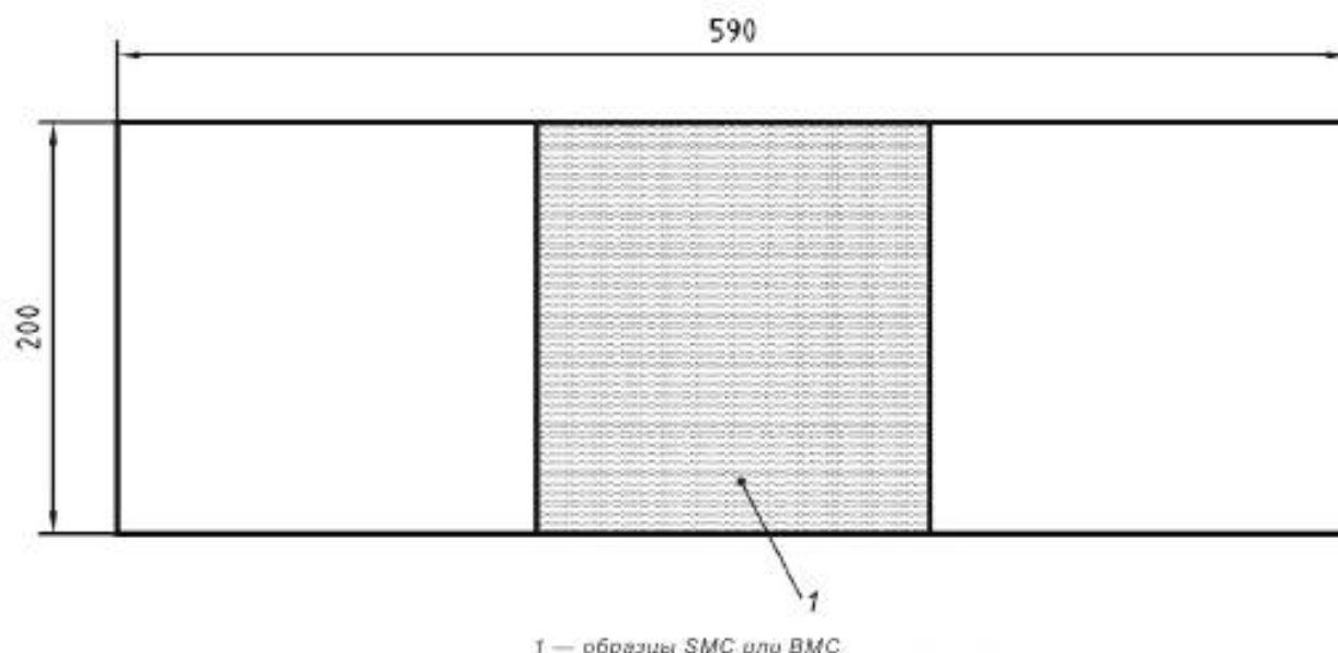
Рисунок 1 — Схема размещения образца в форме при изготовлении пластин по методу В
