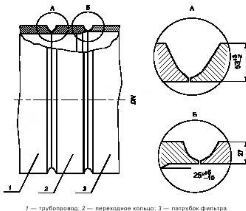
Рисунок 5 — Пример соединения патрубка фильтра с трубопроводом при помощи переходного кольца
