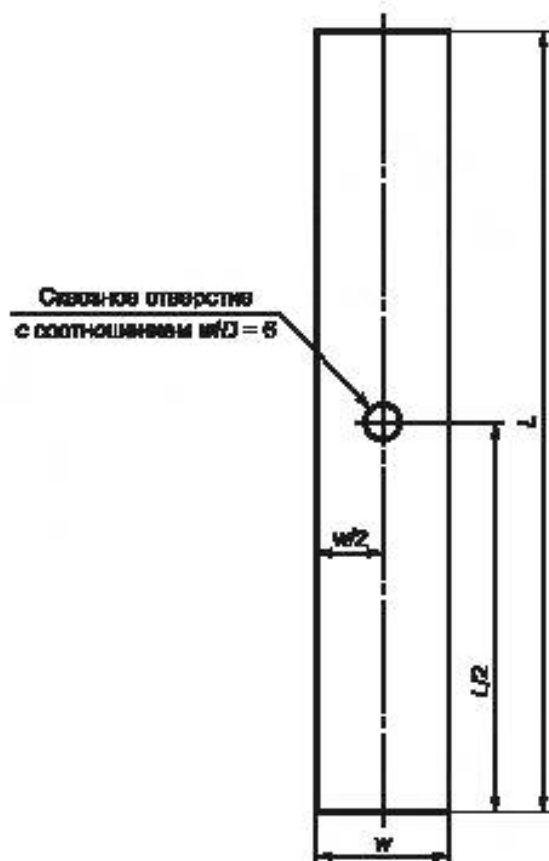
Рисунок 1 — Образец ПК с открытым отверстием для испытаний на растяжение
