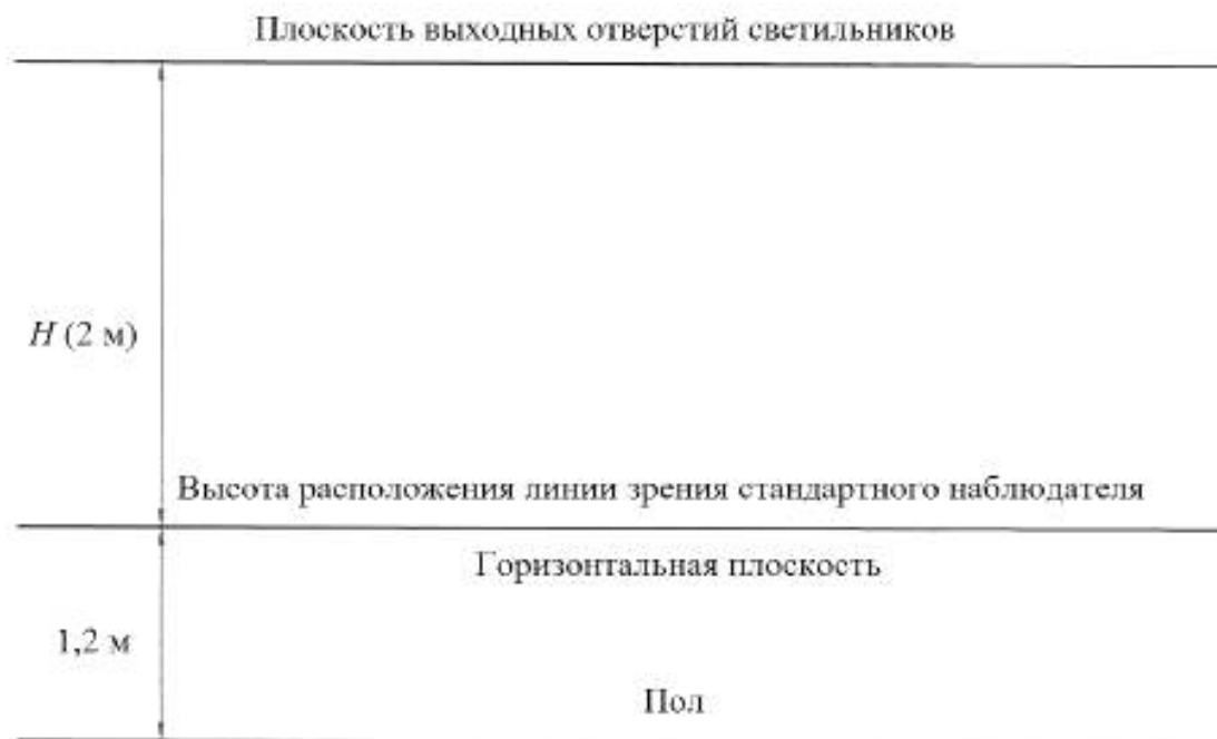
Рисунок 4 — Размеры стандартного модуля в разрезе
