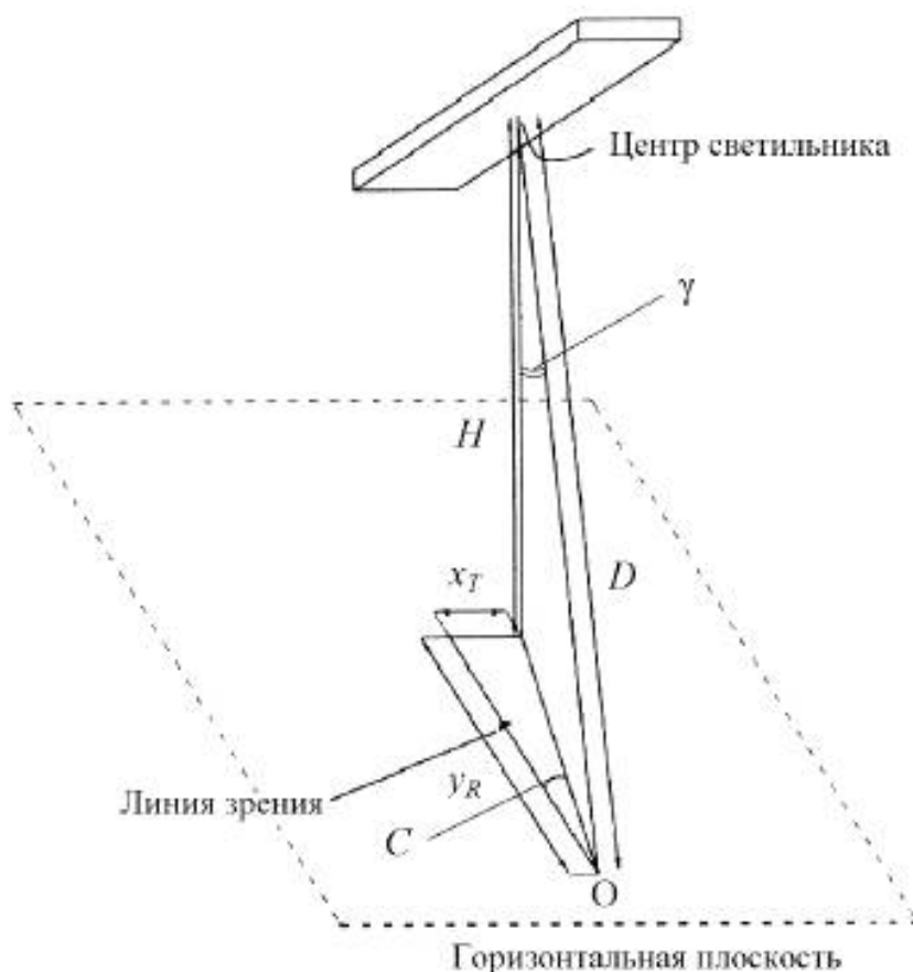
Рисунок 1 — Расположение центра светильника относительно стандартного наблюдателя по [3]
