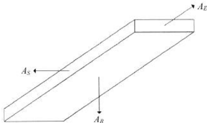
Рисунок 2 — Расположение светящихся поверхностей светильника, видимых стандартному наблюдателю
