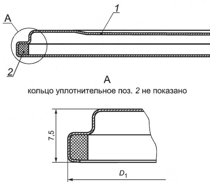
Рисунок 1 — Крышка типоразмеров I-58, I-82
