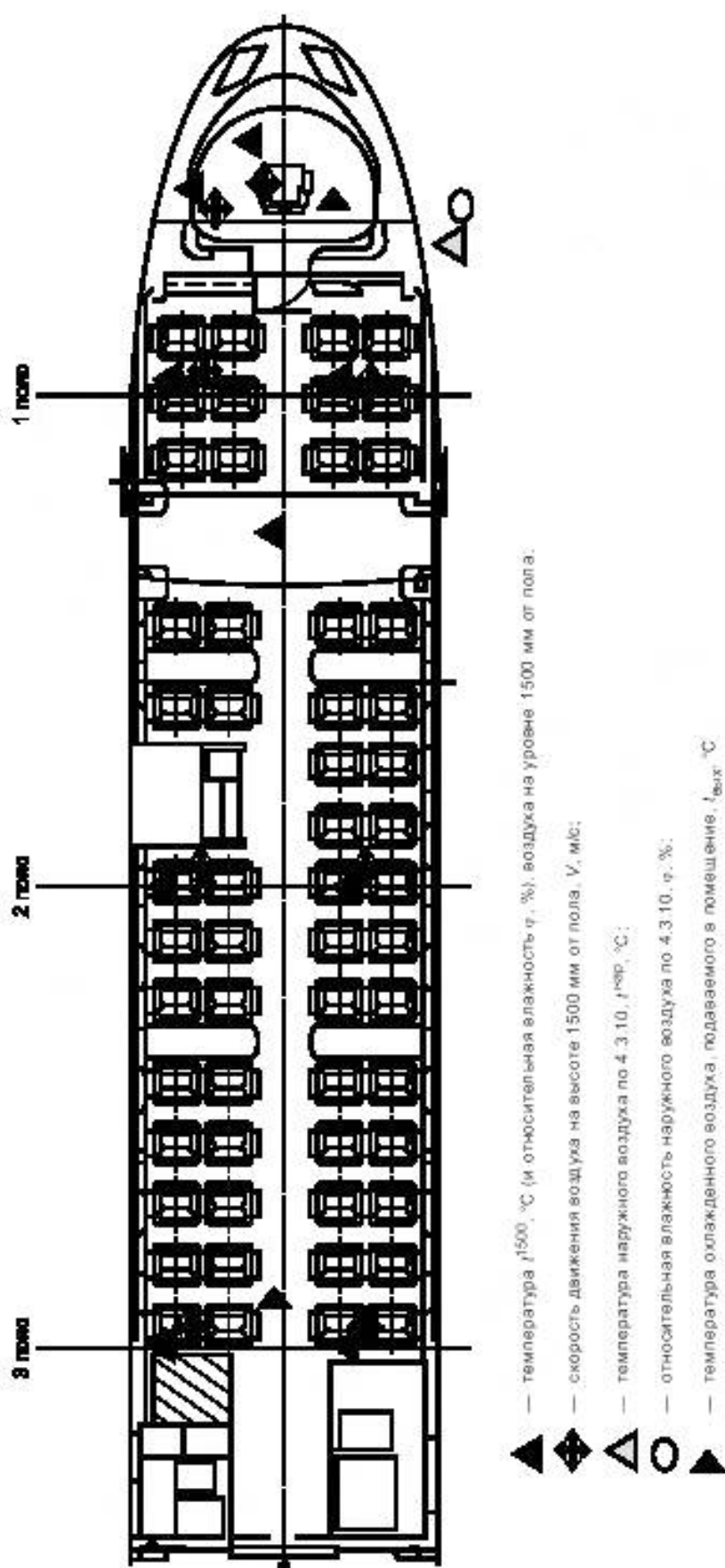
Рисунок Б.1 — Размещение точек измерения параметров микроклимата для теплого периода года в салоне головного вагона
