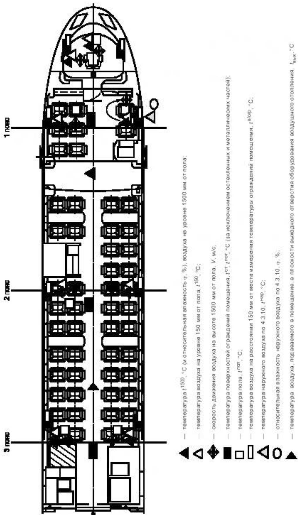
Рисунок Б.7 — Размещение точек измерения параметров микроклимата для холодного периода года в салоне головного вагона
