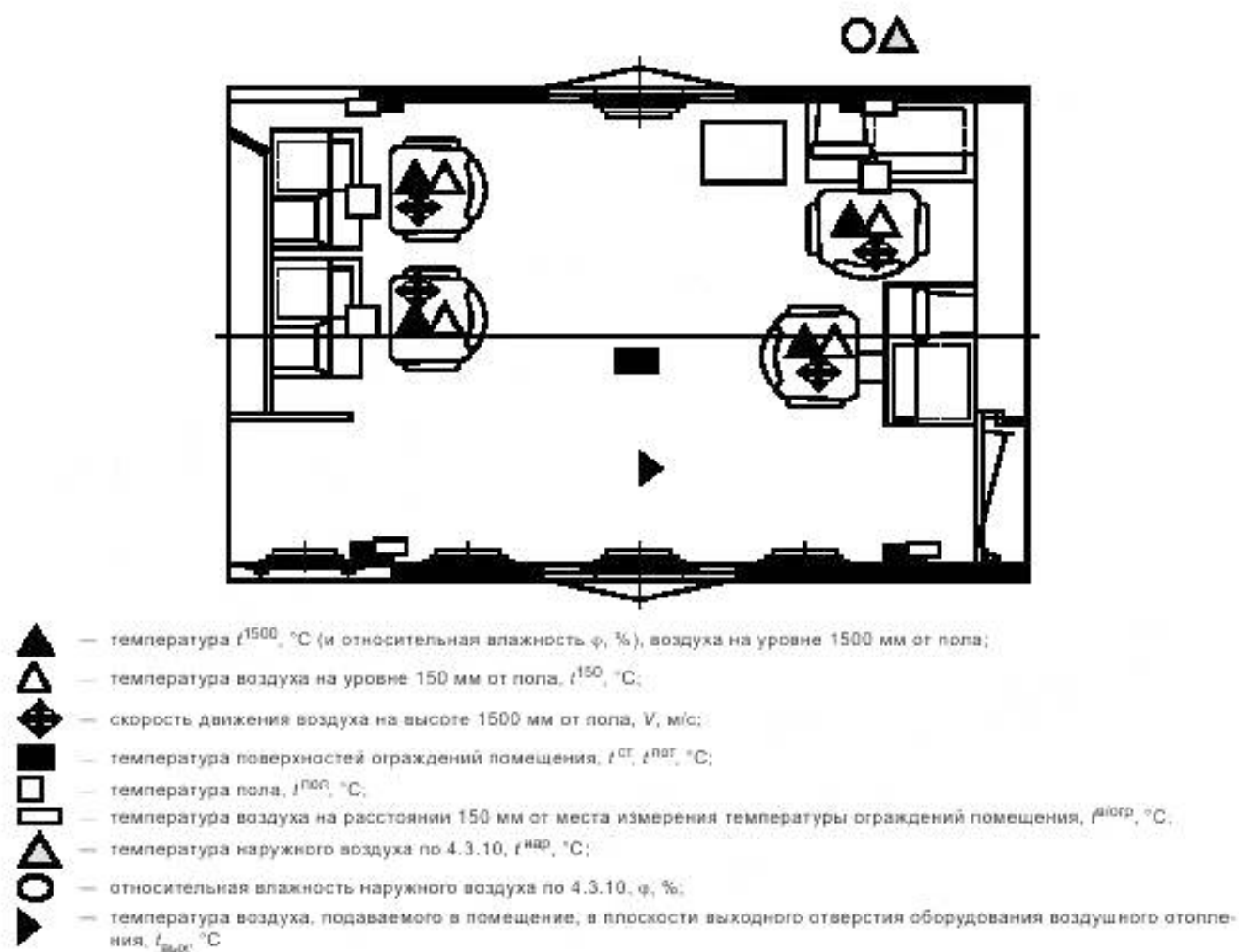
Рисунок Б.11 — Размещение точек измерения параметров микроклимата для холодного периода года в операторской СПС
