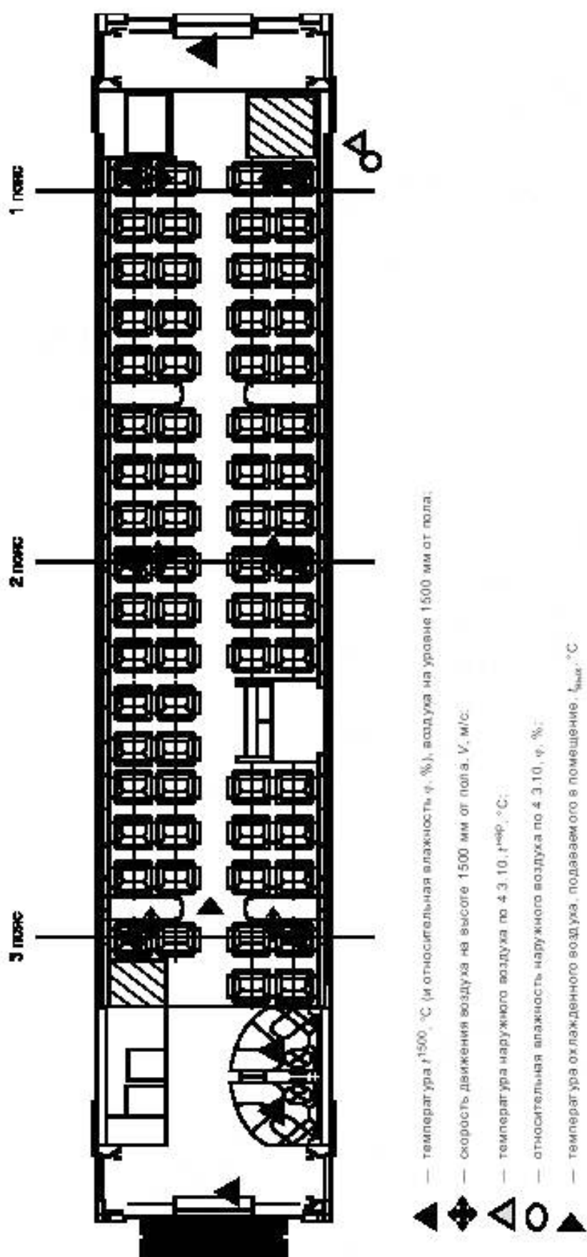
Рисунок Б.2 — Размещение точек измерения параметров микроклимата для теплого периода года в салоне прицепного вагона
