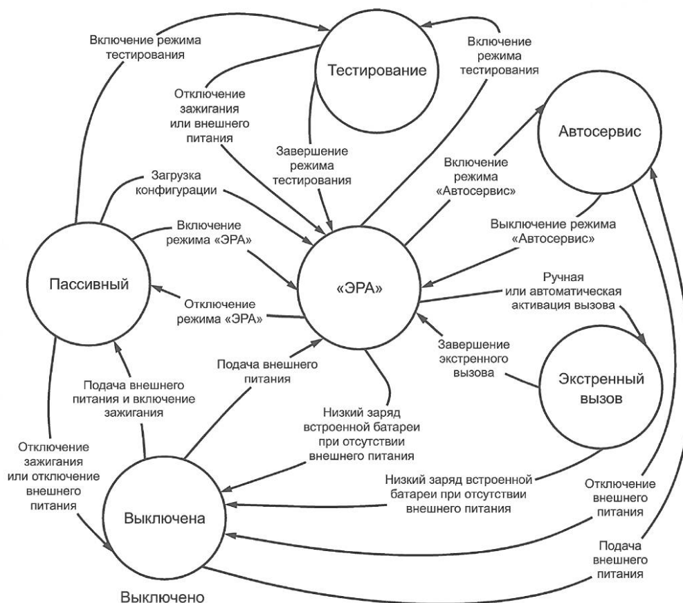
Рисунок 1— Диаграмма состояний устройства/системы вызова экстренных оперативных служб в конфигурации ДО
