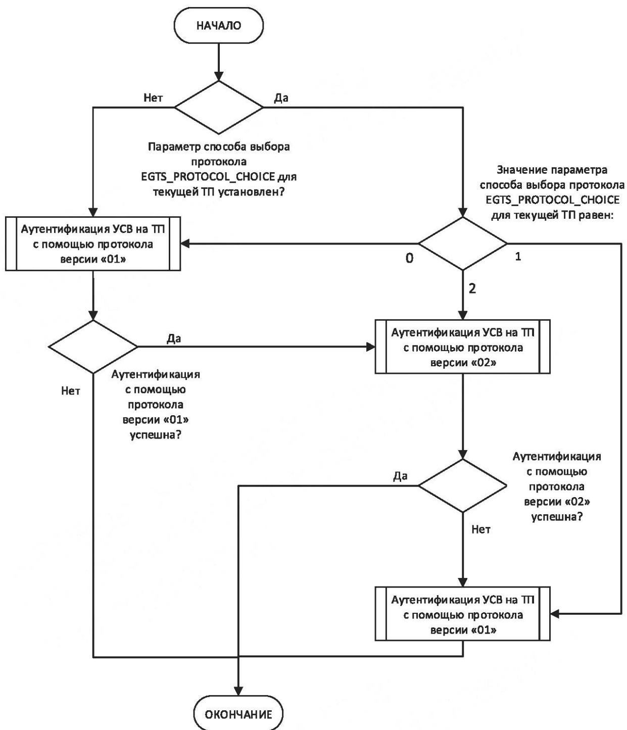
Рисунок 11 — Алгоритм выбора версии протокола при авторизации UCSB на стороне ТП
