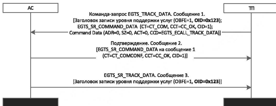
Рисунок 6 — Алгоритм способа использования OID
