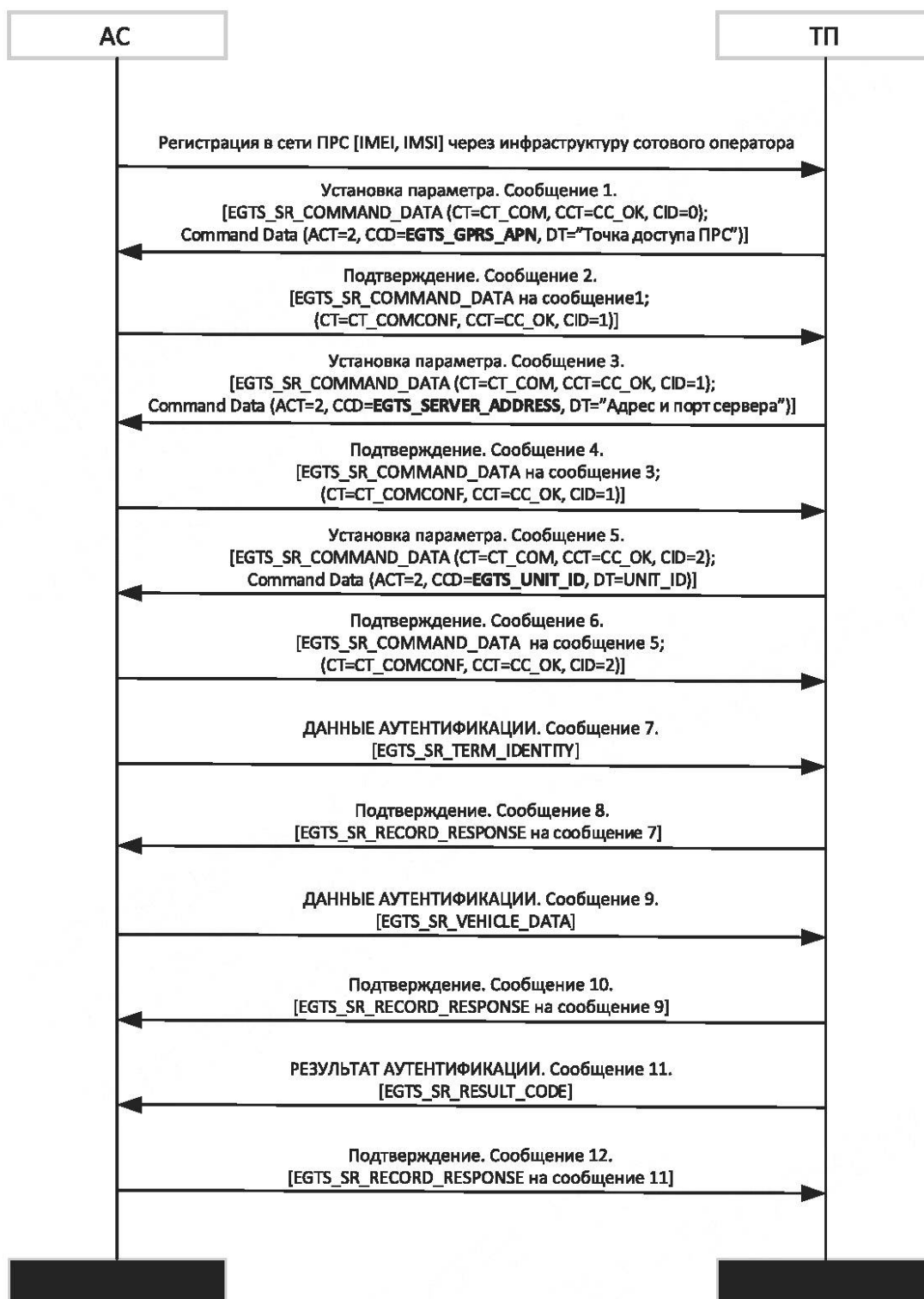
Рисунок 8 — Алгоритм конфигурации UCB с использованием SMS
