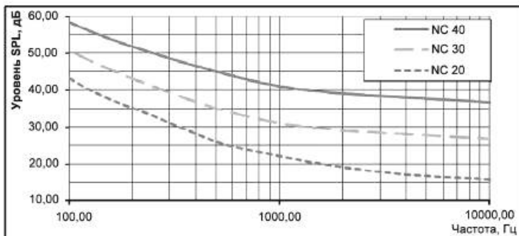
Рисунок 4 — Спектральная плотность окружающего шума
