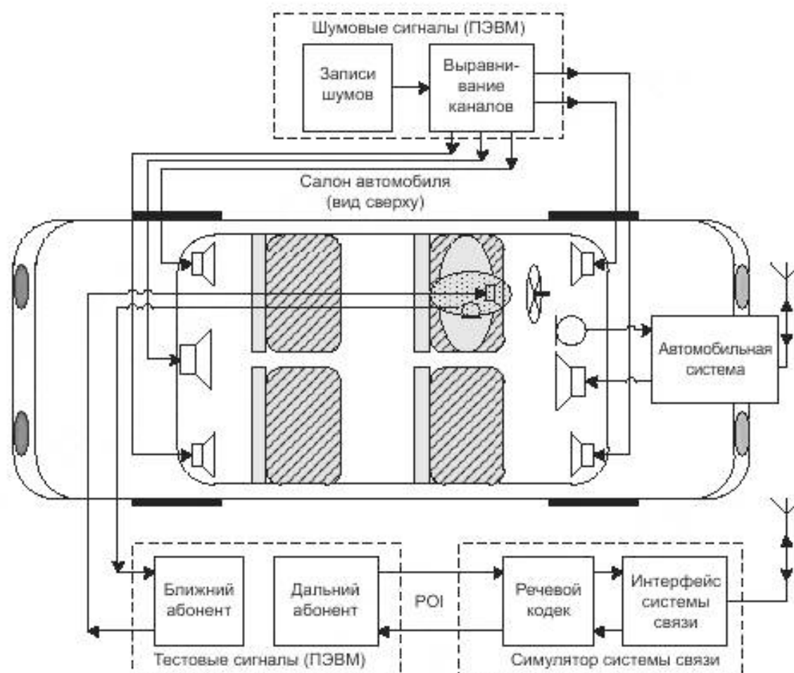
Рисунок 3 — Тестовое оборудование для имитации внешнего акустического шума
