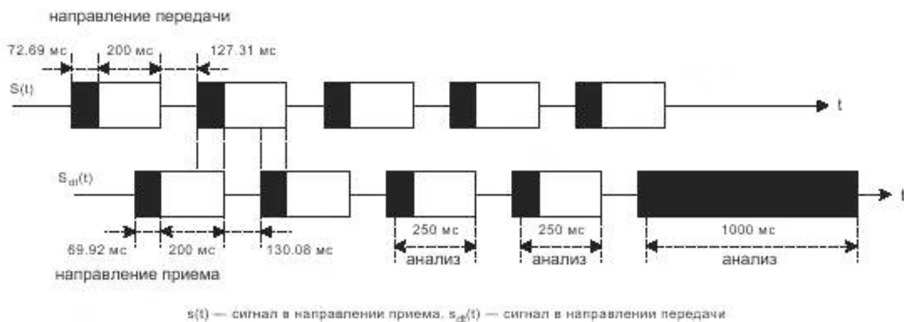
Рисунок 13 — Тестовые сигналы для определения диапазона затухания в направлении приема во время одновременного разговора
