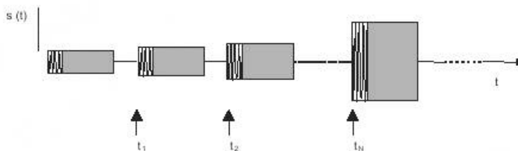
Рисунок 10 — Тестовый сигнал для определения минимального уровня активации и времени включения канала [10]
