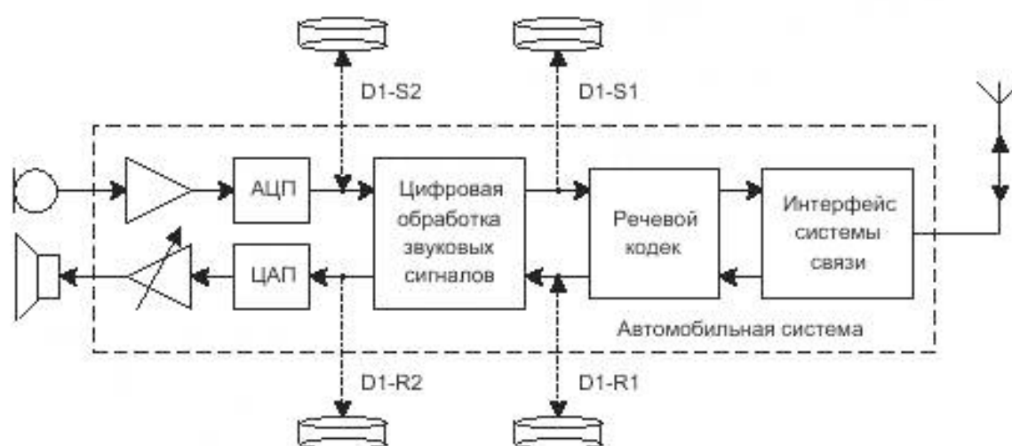
Рисунок В.1 — Отладочный цифровой интерфейс
