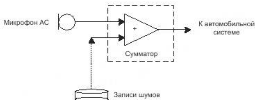
Рисунок Б.1 — Блок-схема электрического способа подмешивания предварительно записанных шумов к тестовым сигналам
