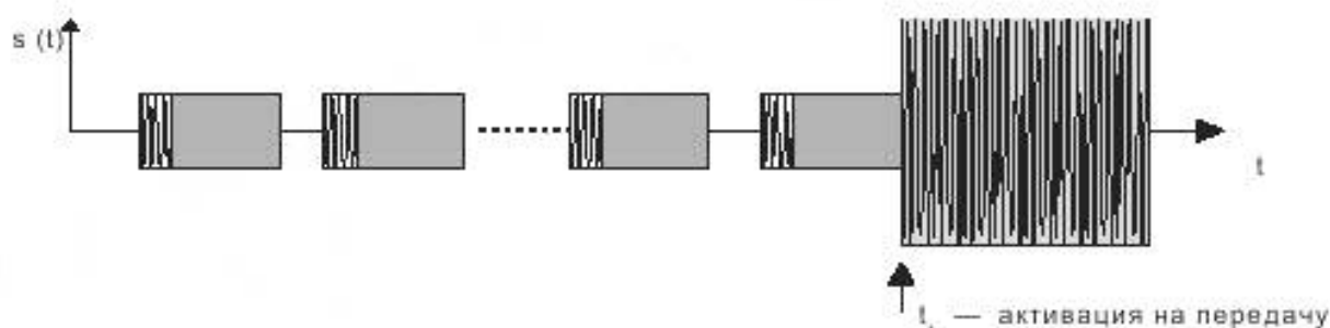
Рисунок 11 — Временная диаграмма сигналов для измерения затухания в канале передачи [10].
