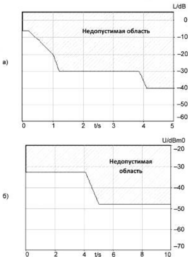
Рисунок 8 — Зависимость степени подавления эхосигналов L и уровня эхосигналов U от времени
