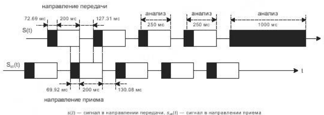
Рисунок 12 — Тестовые сигналы для определения диапазона затухания в направлении передачи во время одновременного разговора
