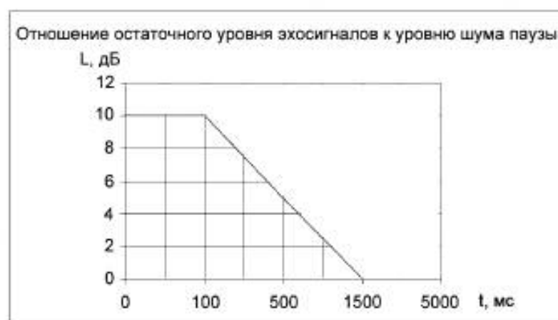
Рисунок 9 — Зависимость отношения остаточного уровня эхосигналов к уровню шума паузы от времени
