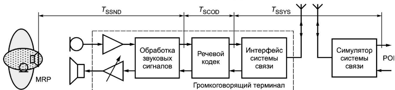
Рисунок 6 — Задержка распространения сигнала в канале передачи
