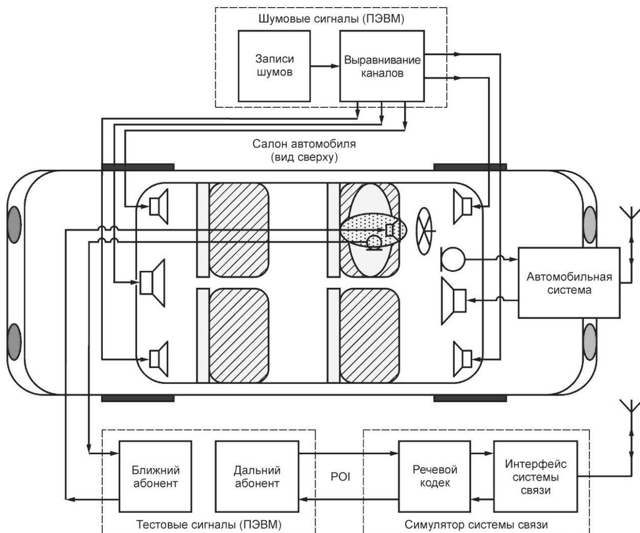
Рисунок 3 — Тестовое оборудование для имитации внешнего акустического шума
