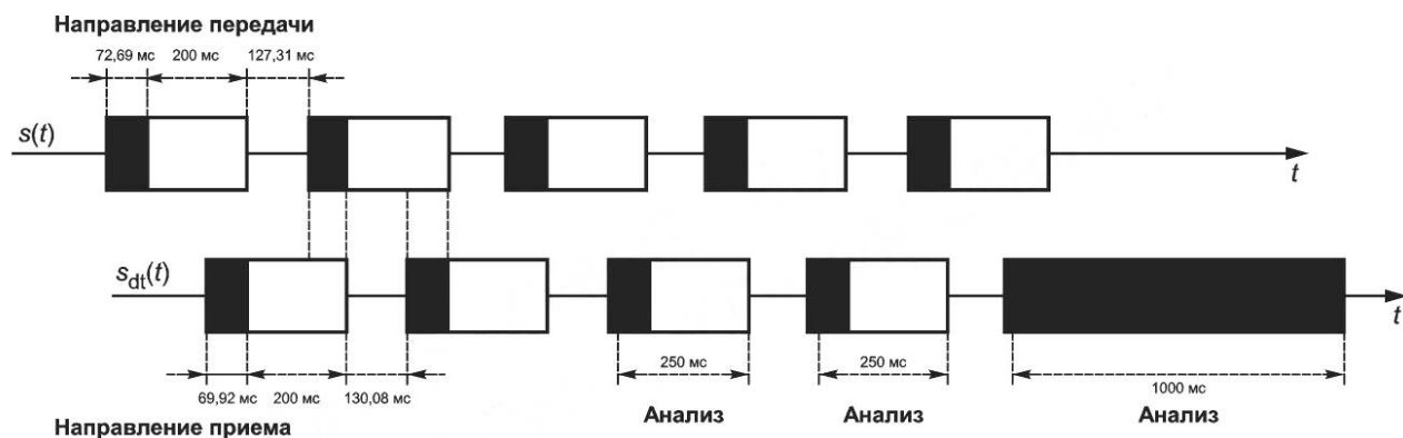
Рисунок 12 — Тестовые сигналы для определения диапазона затухания в направлении приема во время одновременного разговора
