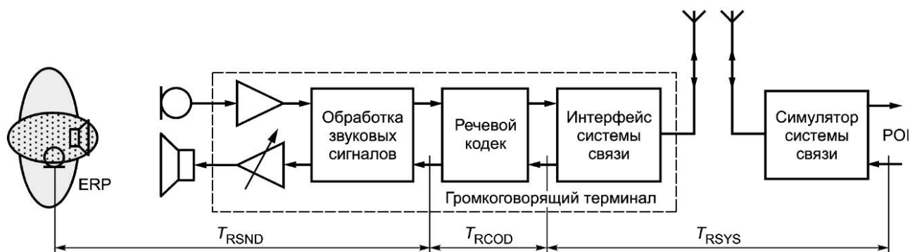
Рисунок 7 — Задержка распространения сигнала в направлении приема
