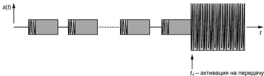
Рисунок 10 — Временная диаграмма сигналов для измерения затухания в канале передачи [10]
