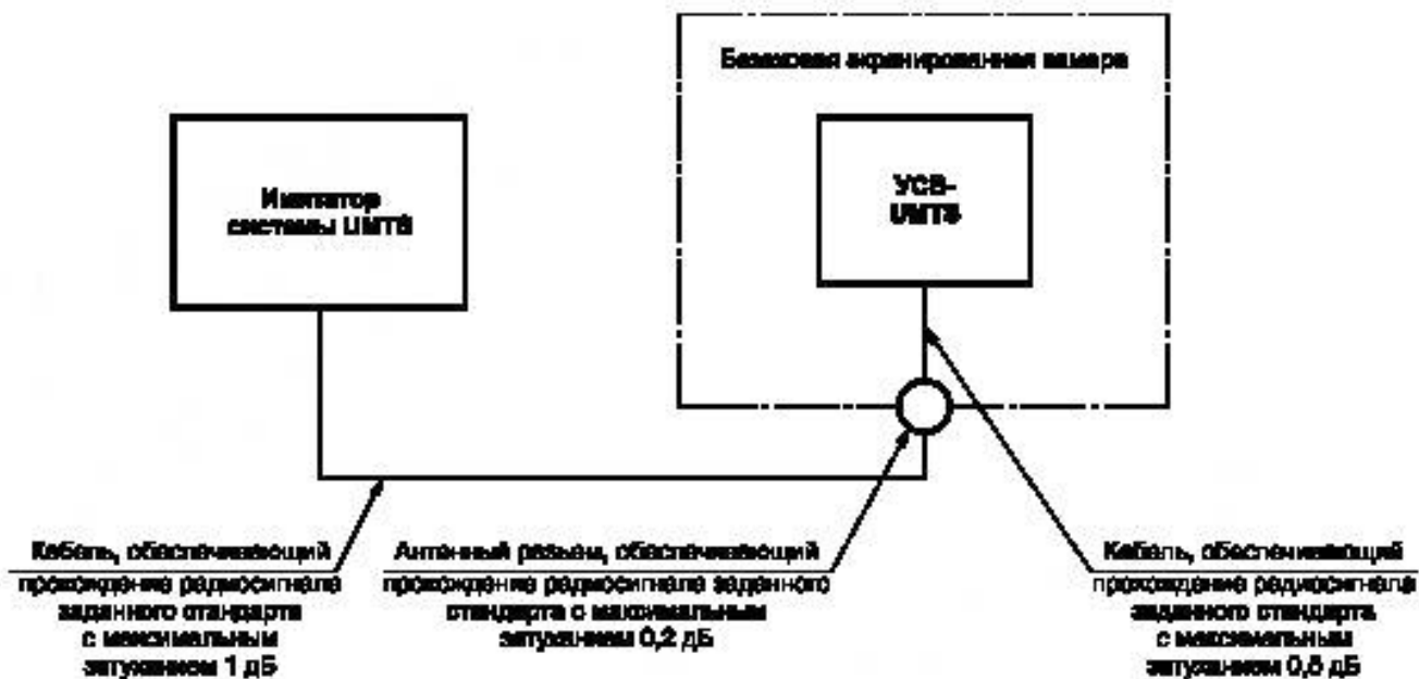
Рисунок Д.1 — Схема испытаний UCS-UMTS с использованием имитатора системы UMTS
