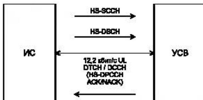
Рисунок Д.2 — Схема испытаний UCS-UMTS для определения предельно допустимой максимальной мощности в режиме HSDPA
