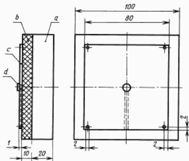
a — квадратная пластина из твердой древесины; b — материал тепловой изоляции: этот материал не должен быть сжат между медной пластиной и пластиной из твердой древесины; c — квадратная медная пластина; d — термопара, укрепленная в центре медной пластины; проволока термопары пропущена между медной пластиной и материалом тепловой изоляции
