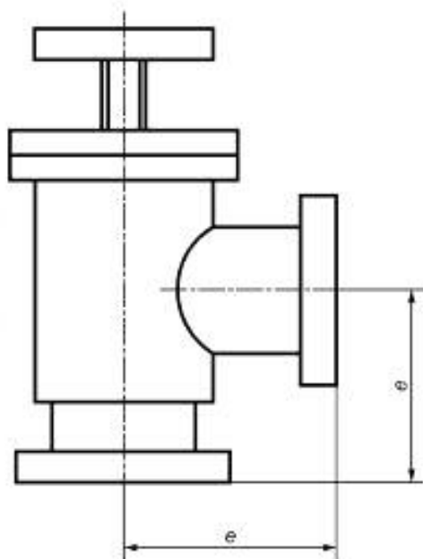
Рисунок 1 — Установочные размеры вакуумных соединений углового клапана
