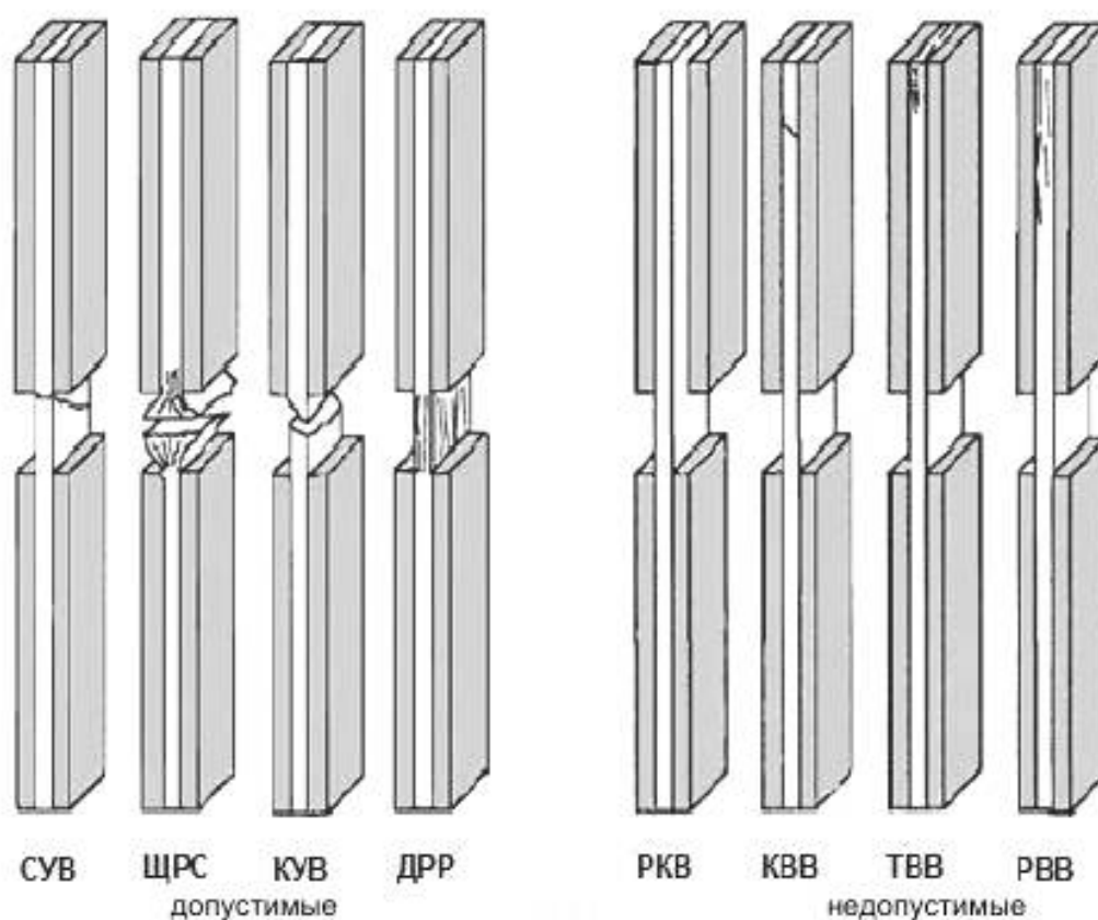
Рисунок 4 — Допустимые и недопустимые типы и области разрушения
