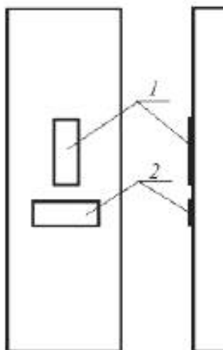
Рисунок 3 — Схема установки экстензометров на образце для определения коэффициента Пуассона при сжатии
