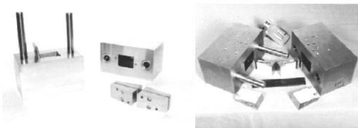
Рисунок Б.2 — Фотографии приспособления для испытаний ПК на сжатие по стандарту [1].
