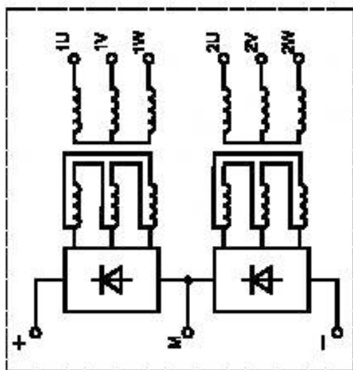
Рисунок 5а — Трехфазное электрооборудование с двумя группами элементов
