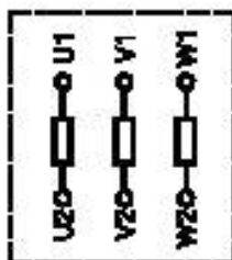
Рисунок 3 — Трехфазное электрооборудование с шестью выводами
