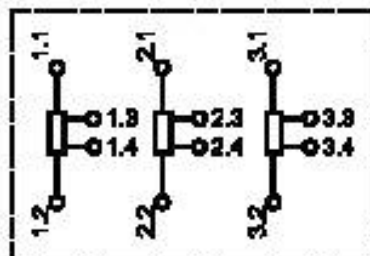
Рисунок 4 — Трехэлементное электрооборудование с двенадцатью выводами: шестью конечными точками и шестью промежуточными точками
