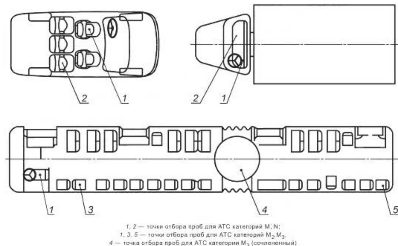
Рисунок Б.1 — Точки отбора проб воздуха и экспресс-анализа ЗВ на месте водителя и пассажирских местах АТС
