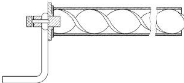
Рисунок 11 — Сверло
