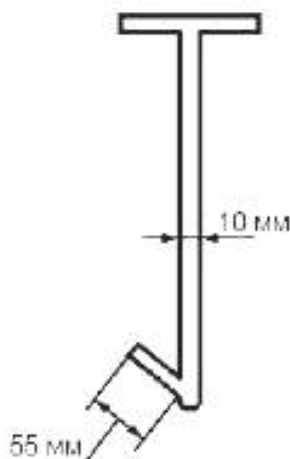
Рисунок 10 — Крюк
