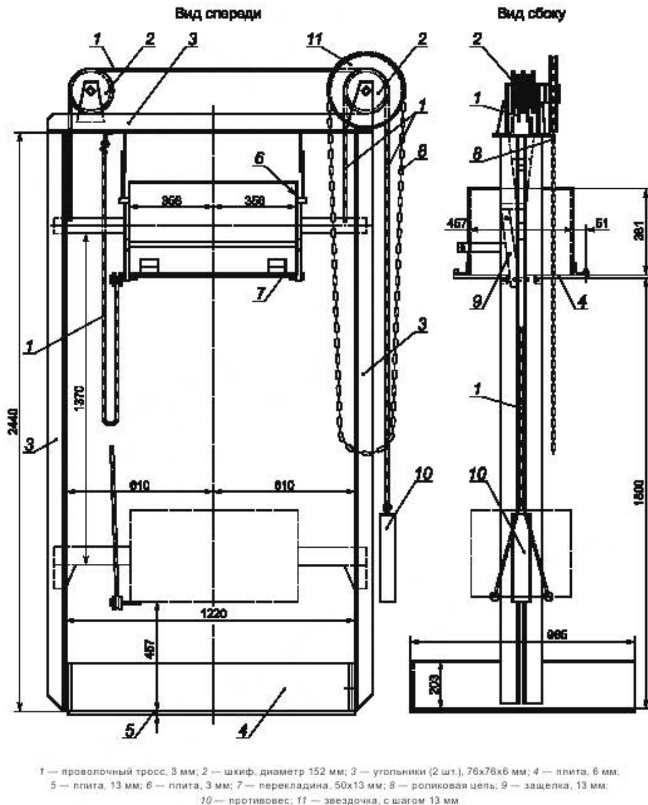
Рисунок 1 — Аппарат для определения прочности на сбрасывание
