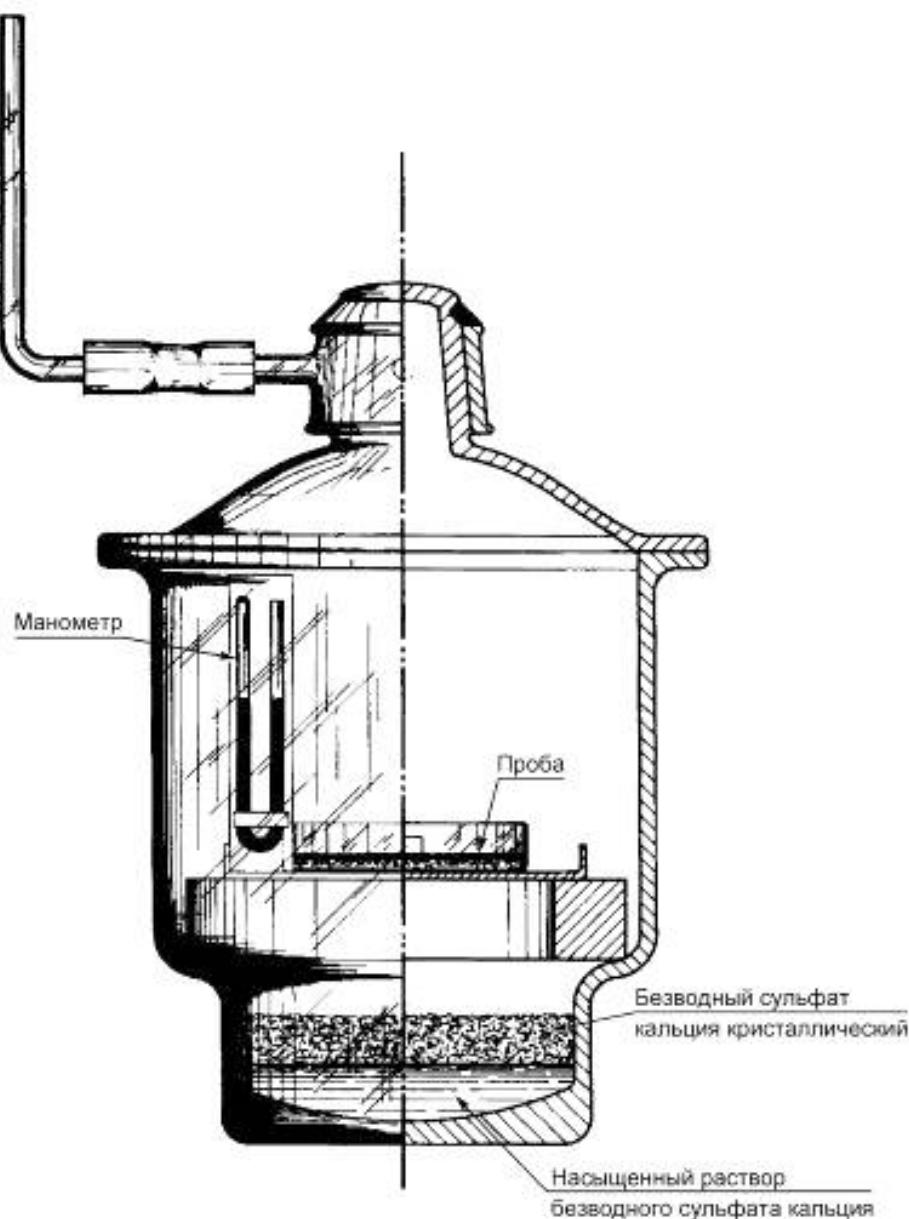
Рисунок 1 — Вакуумный эксикатор
