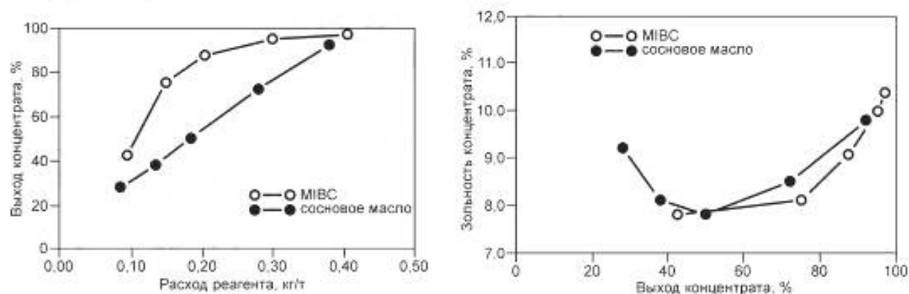
Рисунок А.1 — Пример построения кривых «извлечение/содержание» для углей месторождения Мари Ли
