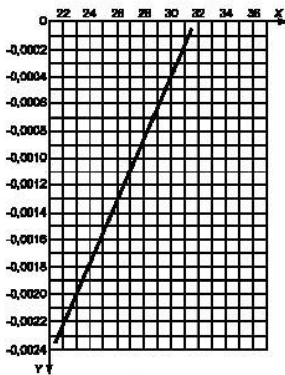
Рисунок 1 — Пример графика составных поправок для ареометра
