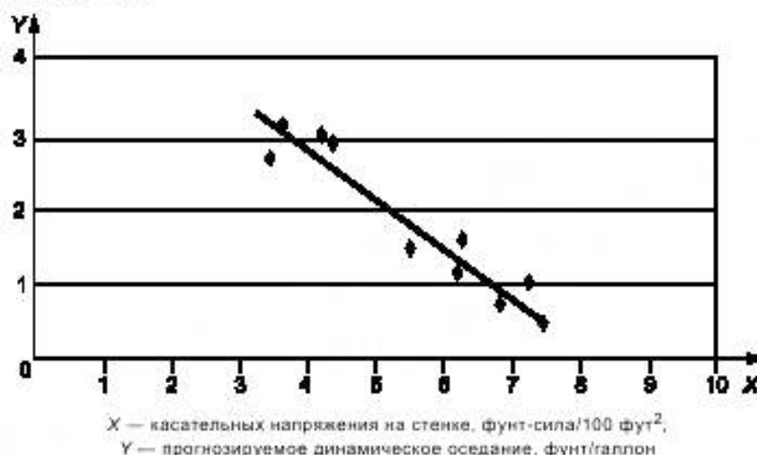
Рисунок О.10 — Прогнозируемое динамическое оседание как функция вычисленных значений \tau_W
