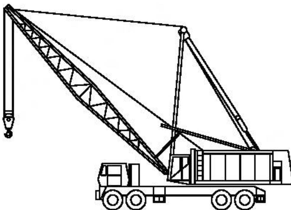
Рисунок 3 — Кран стреловой самоходный с решетчатой (ферменной) стрелой на пневмокопесном шасси, с поворотной верхней конструкцией
