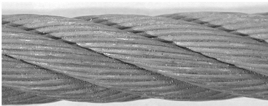
Рисунок Ж.1 — Началo окисления каната (следы коррозии). Коррозию можно удалить протиркой. Степень повреждения — 0 %
