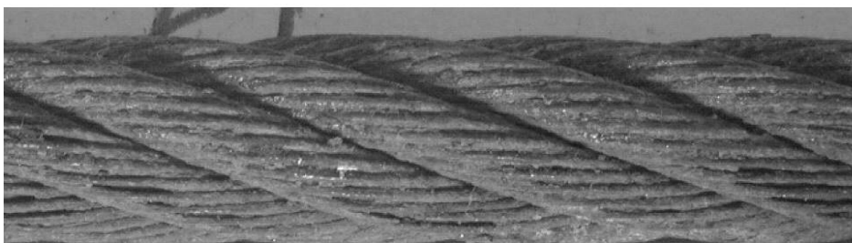
Рисунок Ж.4 — Поверхность проволок сильно поражена точечной коррозией, язвочки на проволочках, ослабленные проволочки, просветы между проволочками. Степень повреждения — 100 % — выбраковка каната
