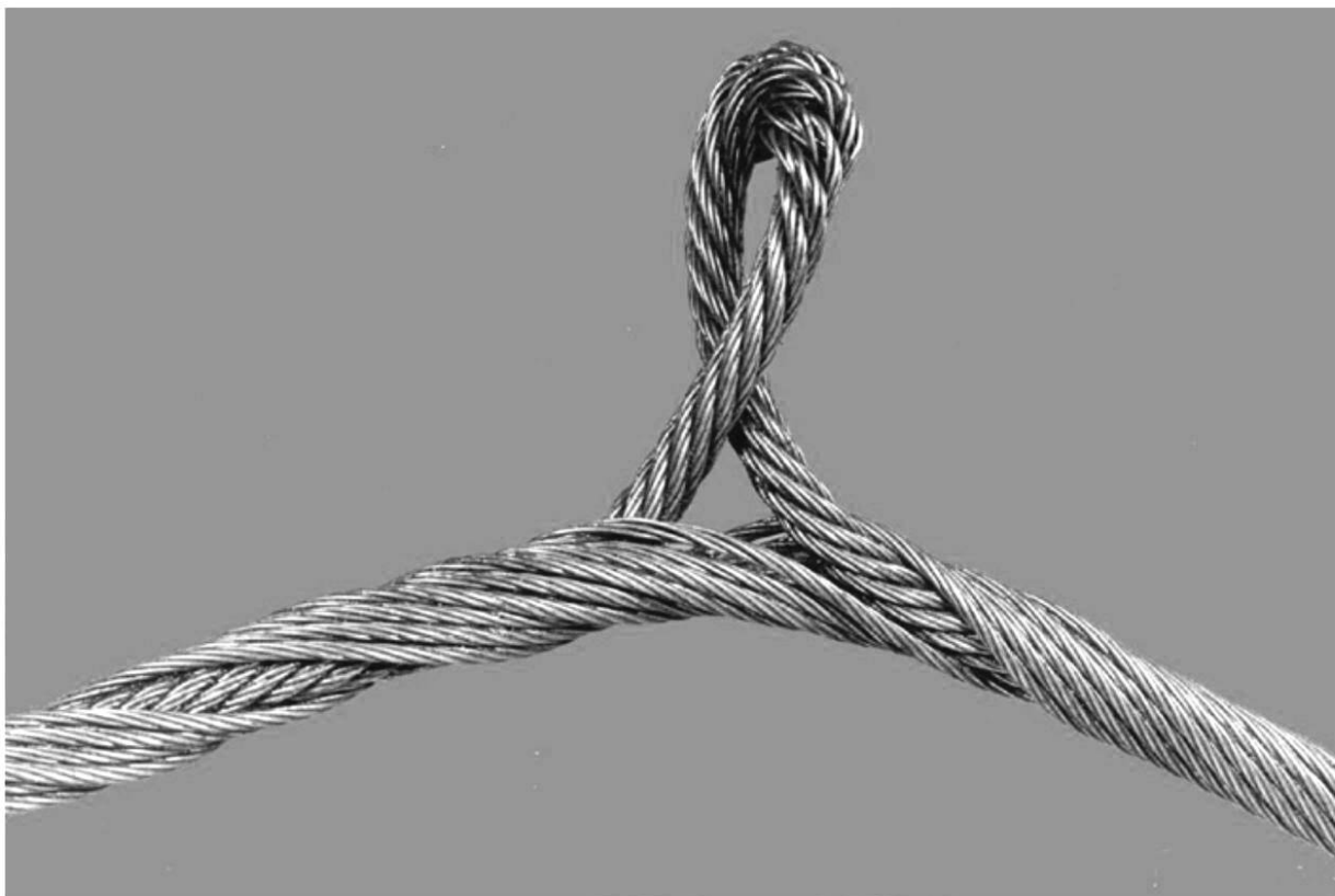
Рисунок А.15 — Некрутящийся канат с выдавленной внутренней частью
