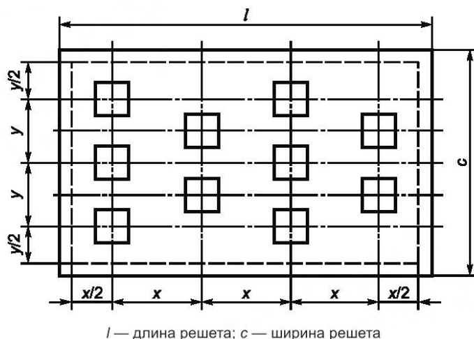
Рисунок Д.1 — Образец нанесения квадратов при определении степени забиваемости отверстий решет
