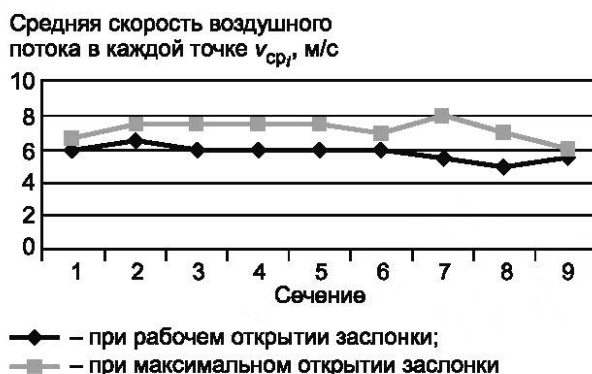
Рисунок В.1 — График результатов измерения скорости воздушного потока в рабочем канале зерноочистительной машины
