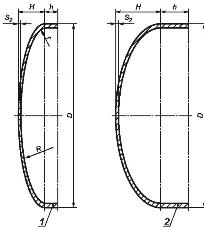
1 — торосферическое днище; 2 — эллиптическое днище
