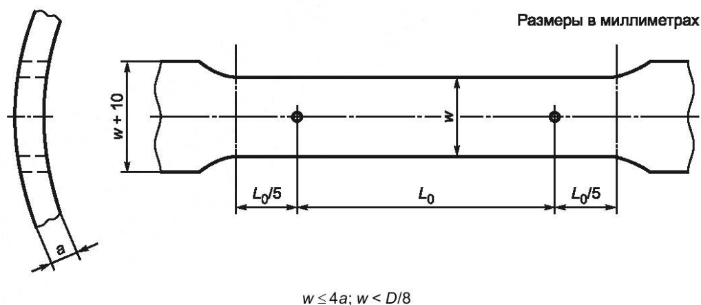
Рисунок 6 — Образец для испытания на растяжение
