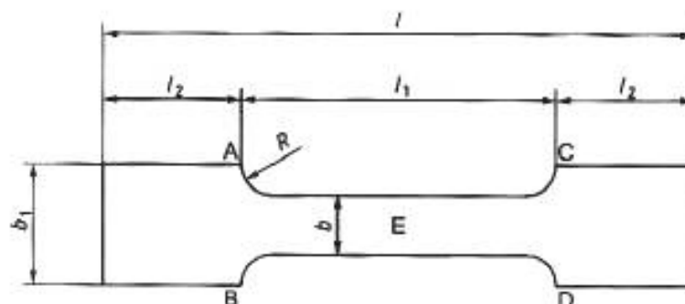
Рисунок 1— Форма испытываемого образца
