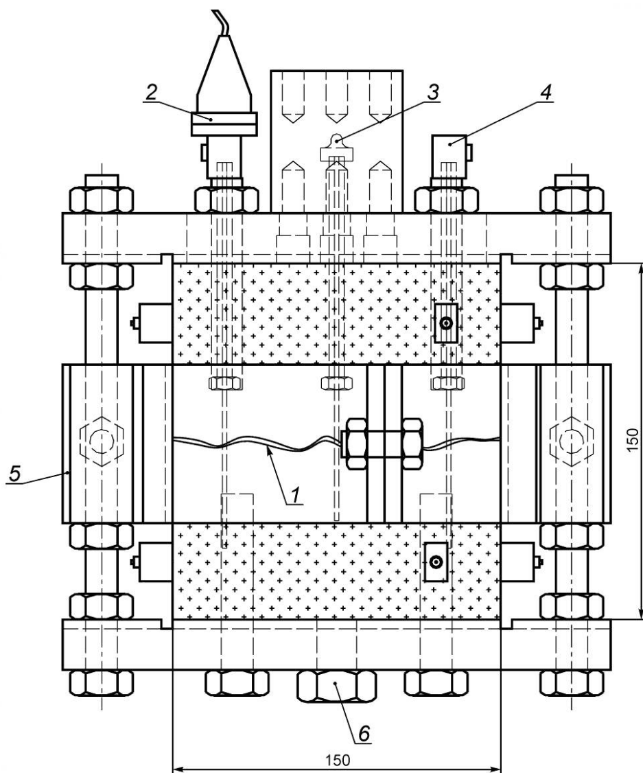
1 — трещина; 2 — датчик давления; 3 — инъекционная головка; 4 — трубка для отвода воздуха (воды); 5 — обойма и резиновый жгут; 6 — винт М24 (позиция 9 по таблице П.1)
