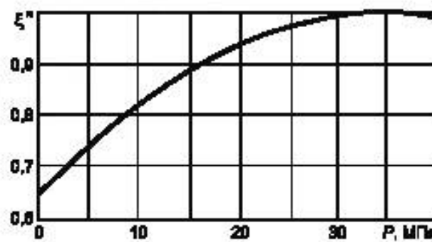
Рисунок 8 — Поправочные коэффициенты \xi' и \xi''
