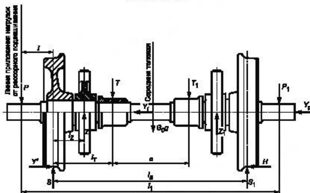
Рисунки А.1 и А.2: T(T_1) — вертикальная сила от опорно-осевого подшипника; P(P_1) — вертикальная нагрузка на буксовую шейку оси со стороны набегающего (сбегающего) колеса; S(S_1) — вертикальная нагрузка на набегающее (сбегающее) колесо от рельса; Z(Z_1) — вертикальная сила на ось от ведомой шестерни; H — поперечная составляющая силы трения внутреннего колеса о рельс; Y — боковая сила рельса на набегающее колесо; Y_i — поперечная сила инерции КП; Y_p — рамная сила; l — расстояние от середины буксовой шейки до плоскости круга катания соседнего колеса; l_1 — расстояние между линиями приложения вертикальной нагрузки к буксовым шейкам оси КП; l_2 — расстояние между плоскостями кругов катания КП; l_T — расстояние от плоскости круга катания набегающего колеса до линии действия силы T ; l_Z — расстояние от плоскости круга катания набегающего колеса до линии действия силы Z ; G_0 — масса части оси, заключенной между плоскостями кругов катания колес; g — ускорение силы тяжести; a — расстояние между силами T и T_1 ; a_1 — расстояние от середины тележки до силы T_1 ; a_2 — расстояние между силами T и Z .
