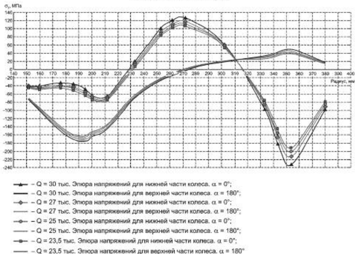
Рисунок Б.6 — Эпюра радиальных напряжений по сечению колеса с его внешней стороны при разных нагрузках Q от КП на рельсы
