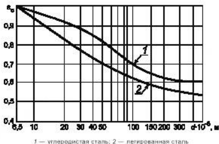
Рисунок 4 — Коэффициенты влияния абсолютных размеров сечения \varepsilon_\sigma на усталостную прочность \beta — коэффициент влияния на предел выносливости качества обработки поверхности (рисунок 5);
