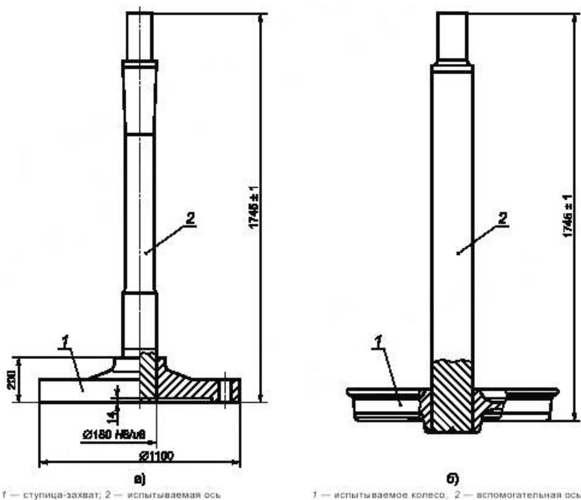
Рисунок И.1 — Образцы сборок для испытаний на усталость полномасштабных оси и колеса
