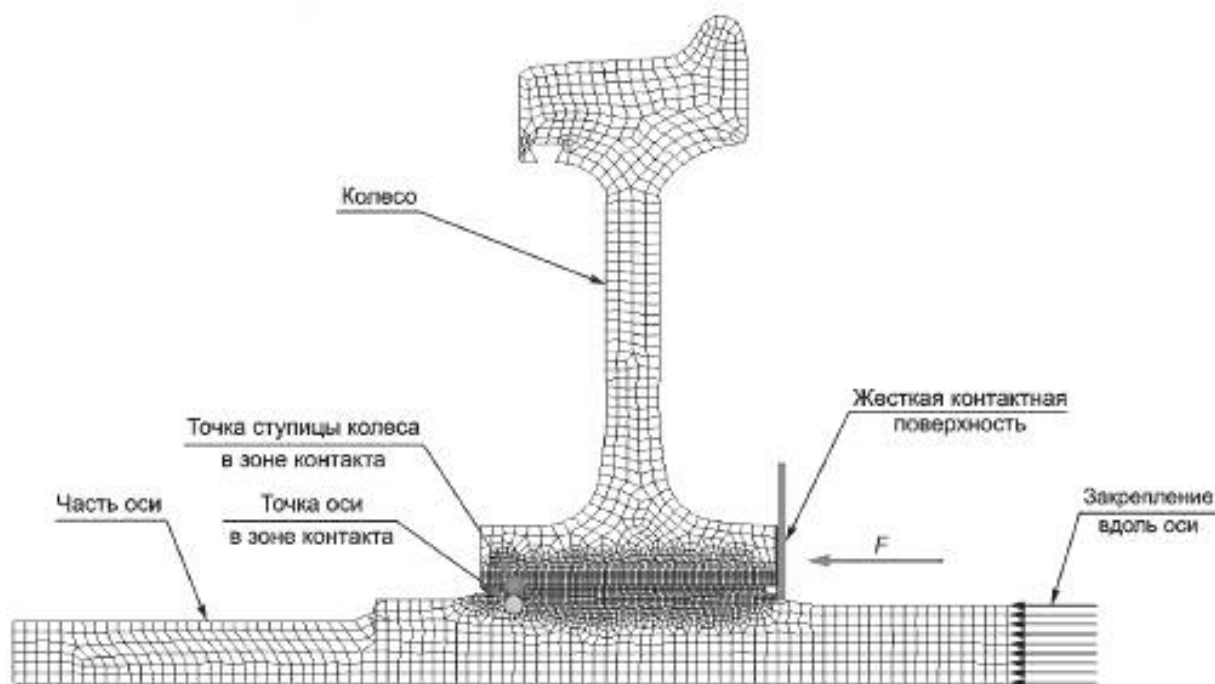
Рисунок Е.1 – Модель колеса и оси, контрольные точки контакта
