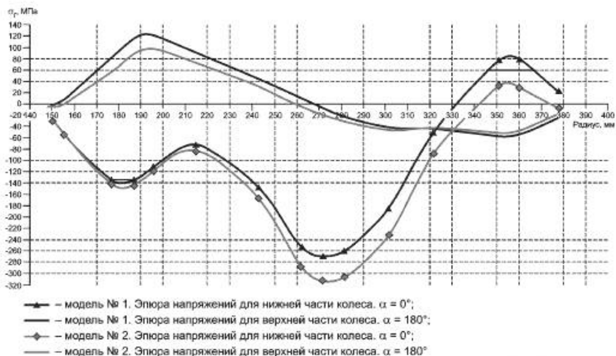
Рисунок Б.3 — Эпюры радиальных напряжений по сечению колеса с полномерным и изношенным ободом с его внутренней стороны при нагрузке от КП на рельсы Q=30 тс ( \Delta=0,25 мм, S=292,6 кН, Y'=90,9 кН)
