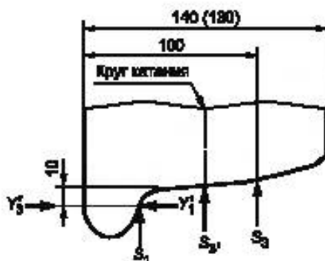
S, Y — вертикальная и боковая нагрузки на набегающее колесо от рельса при режимах: S_1 — движение по кривым участкам пути; S_2 — движение высокоскоростного ПС по специальному пути; S_3 — движение по стрелкам
