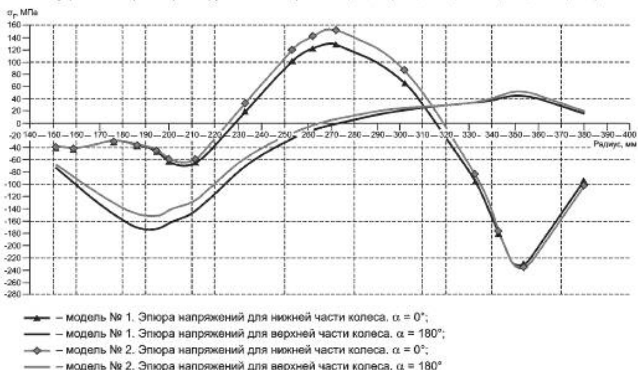
Рисунок Б.4 — Эпюры радиальных напряжений по сечению колеса с полномерным и изношенным ободом с его внешней стороны при нагрузке от КП на рельсы Q=300 кН ( \Delta=0,25 мм, S=292,6 кН, Y'=90,9 кН)
