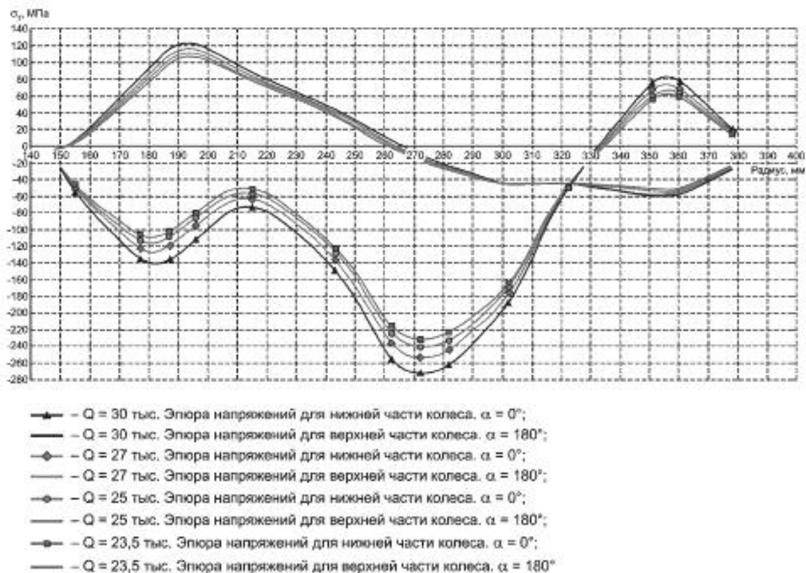
Рисунок Б.5 — Эпюра радиальных напряжений по сечению колеса с его внутренней стороны при разных нагрузках Q от КП на рельсы
