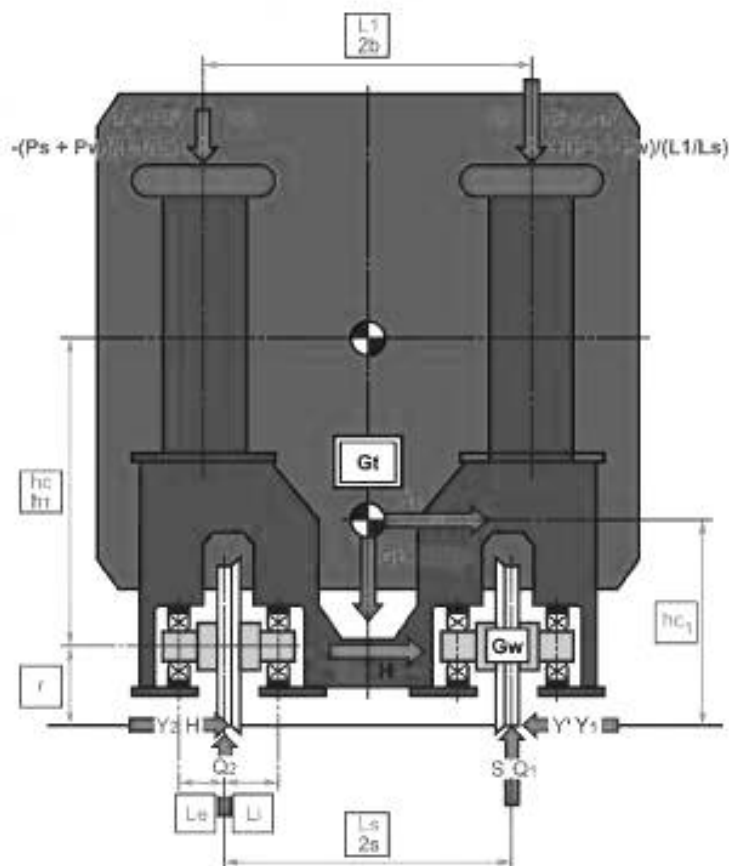
Рисунок А.6 — Схема расположения колесных узлов и действующих нагрузок в экипаже с раздвижной КП
