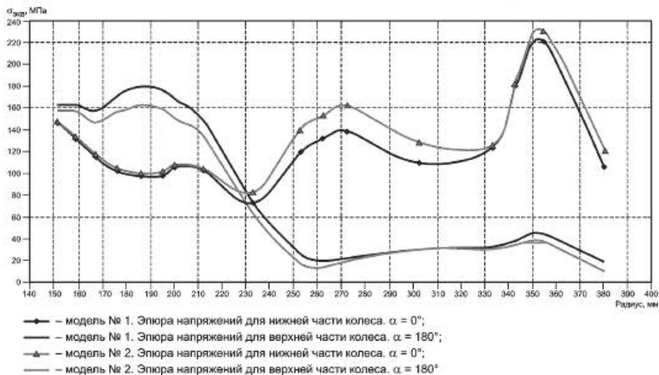
Рисунок Б.2. — Эквивалентные напряжения на внешней стороне колеса
