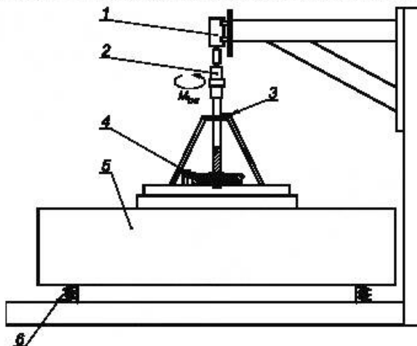
Рисунок Ж.1 — Пример схемы стенов для испытания на усталость колес и осей
