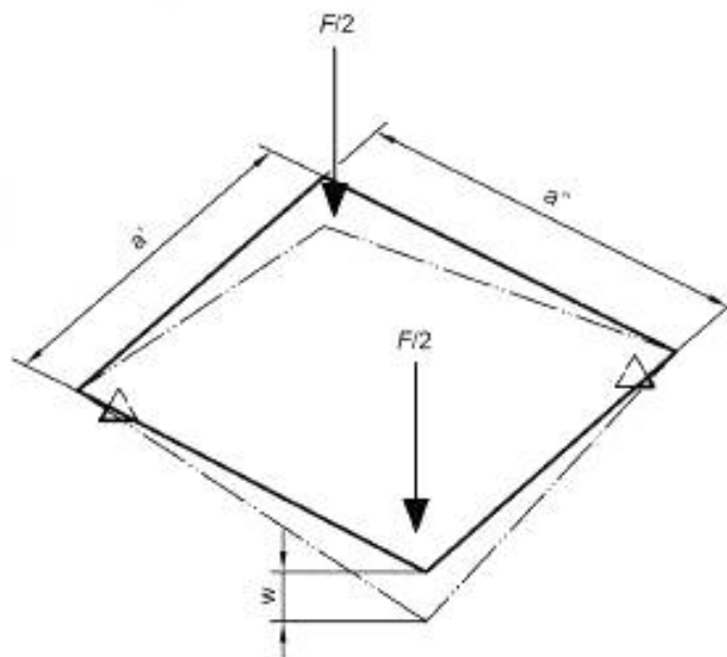
Рисунок 1 — Принцип испытания
