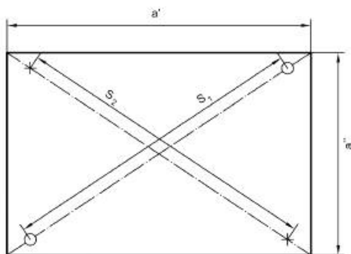
Рисунок 2 — Позиции точек опоры и точек нагружения
