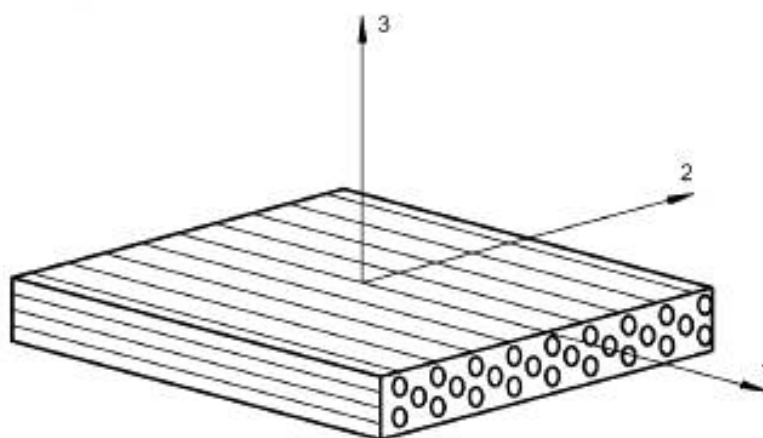
Рисунок 3 — Оси симметрии для материала, армированного волокном
