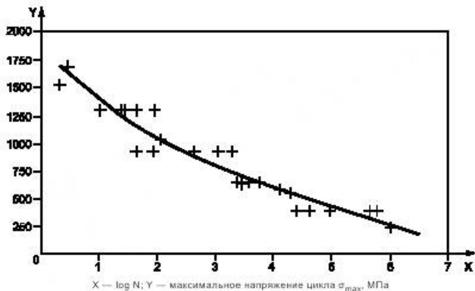
Рисунок 1 — Пример кривой усталости
