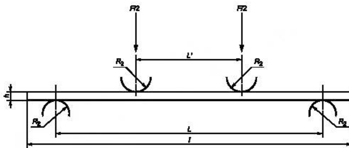
Рисунок ДА.2 — Схема четырехточечного нагружения
