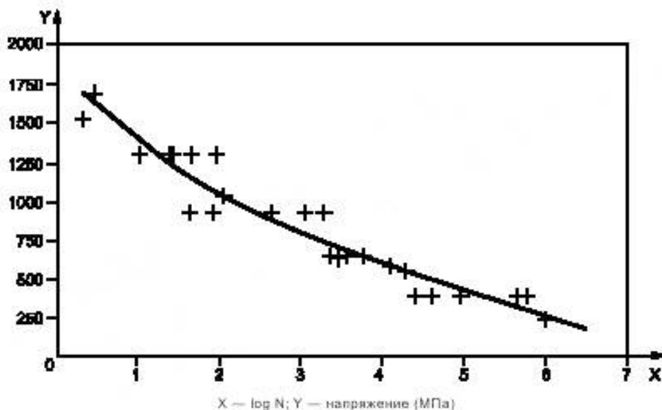
Рисунок 3 —Пример диаграммы усталости
