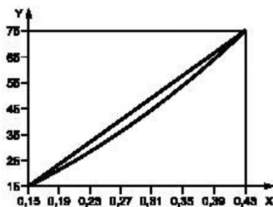
Рисунок А.1 — Типовая петля гистерезиса
