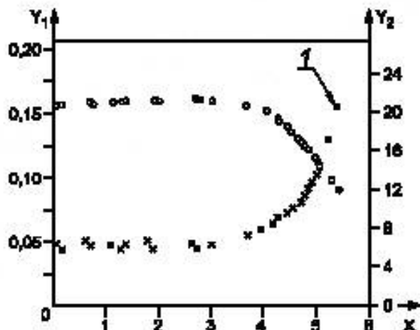
Рисунок А.2 — Динамический модуль упругости и изменение затухания
