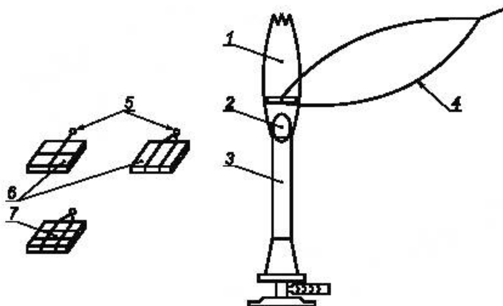
1 — факел пламени; 2 — восстановительная часть пламени; 3 — горелка Бунзена; 4 — пинцет; 5 — нихромовая проволока; 6 — образец, армированный однонаправленными углеродными волокнами; 7 — образец, армированный плетеной тканью из углеродного волокна
