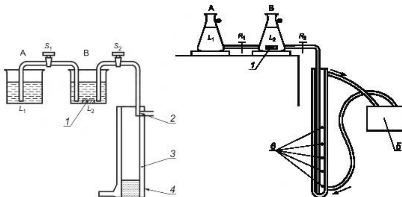
1 — магнитная мешалка; 2 — капилляр касается внутренней поверхности колонки; 3 — колонка; 4 — водная оболочка; 5 — термостат; 6 — калиброванные сферические поплавки
