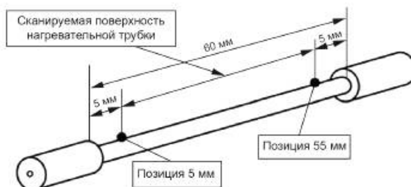
Рисунок А.2.7 — Характеристики сканируемой поверхности нагревательной трубки
