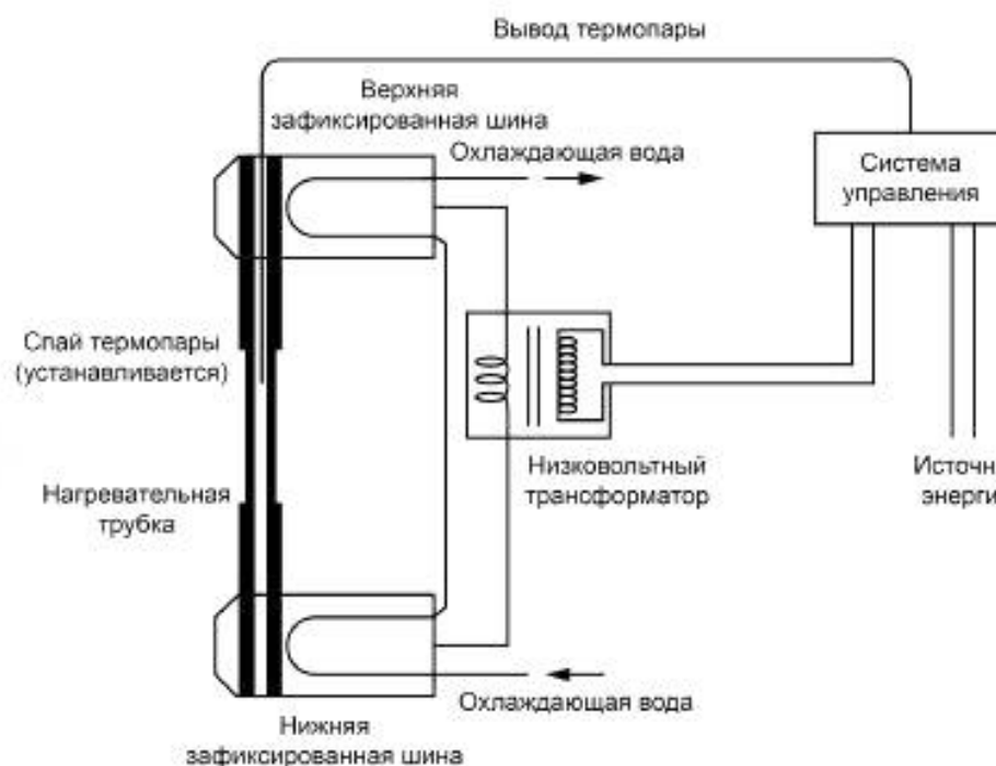
Рисунок А.4.4 — Схема нагревательной трубки и контроля температуры
