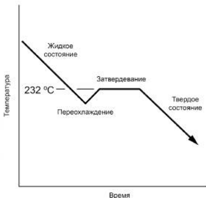
Рисунок А.4.5 — Кривая затвердевания олова
