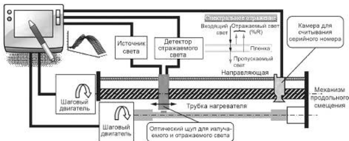
Рисунок A.2.1 — Интерферометр. Общий принцип действия
