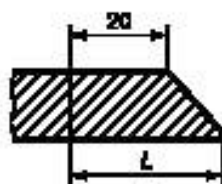
Рисунок 7 — Присоединительный конец под приварку
