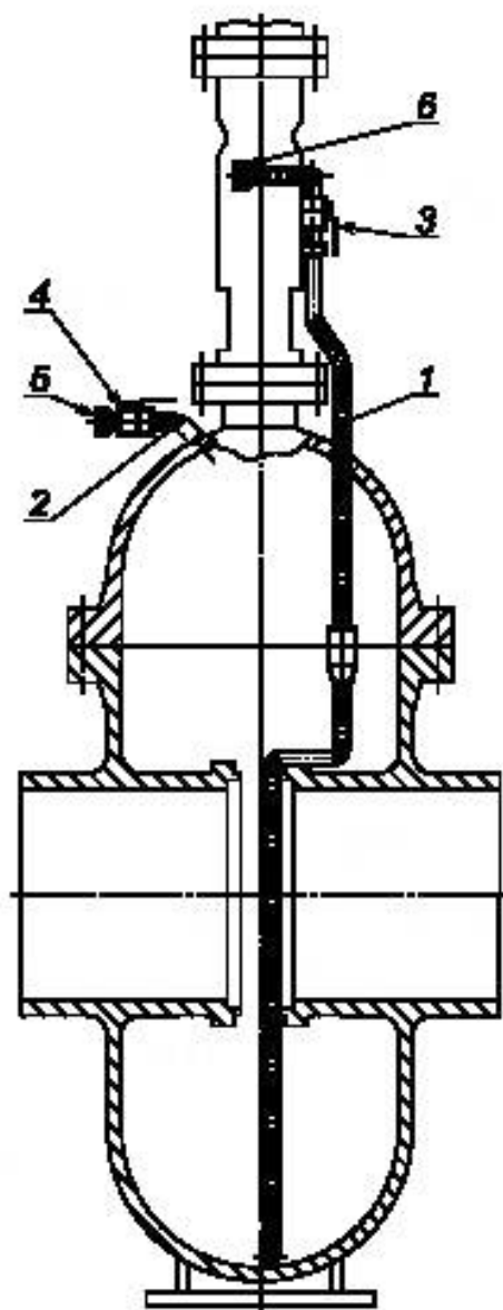
1 — дренажный трубопровод; 2 — спускной трубопровод; 3, 4 — запорная арматура; 5, 6 — заглушка
