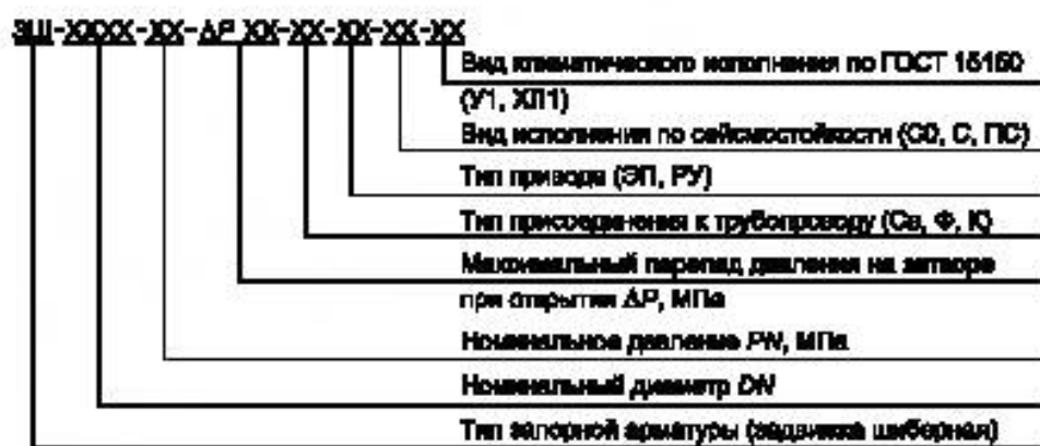
Рисунок 1 — Схема условного обозначения задвижки
