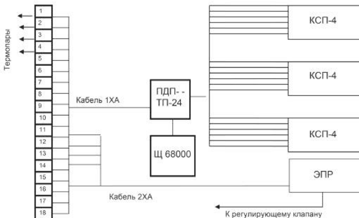
Рисунок 6 — Измерительная схема стенда
